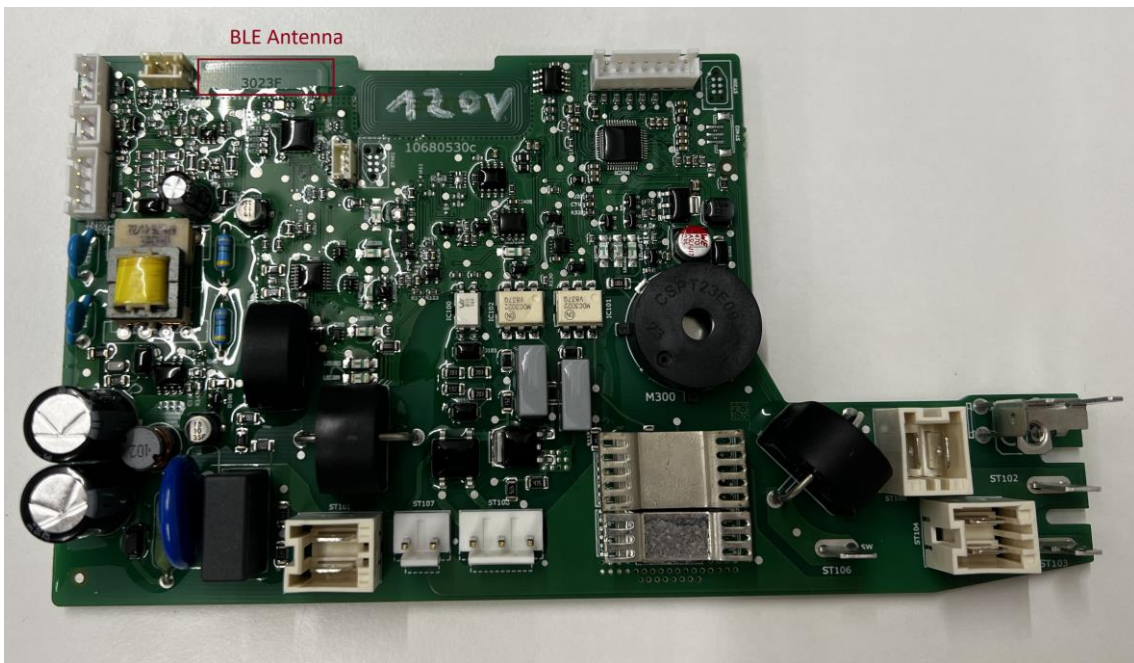
Figure 4: BLE antenna
