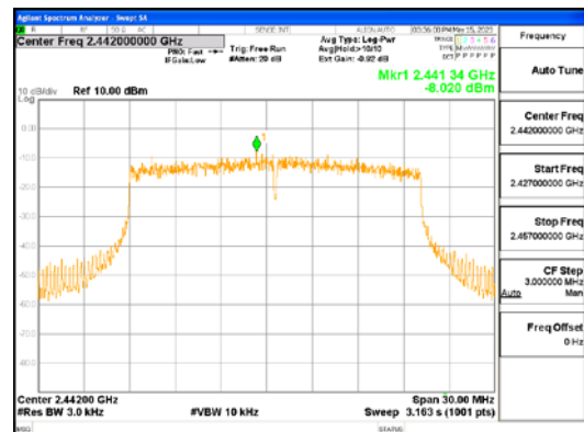
ANT L, 802.11ax_HE20_242T
