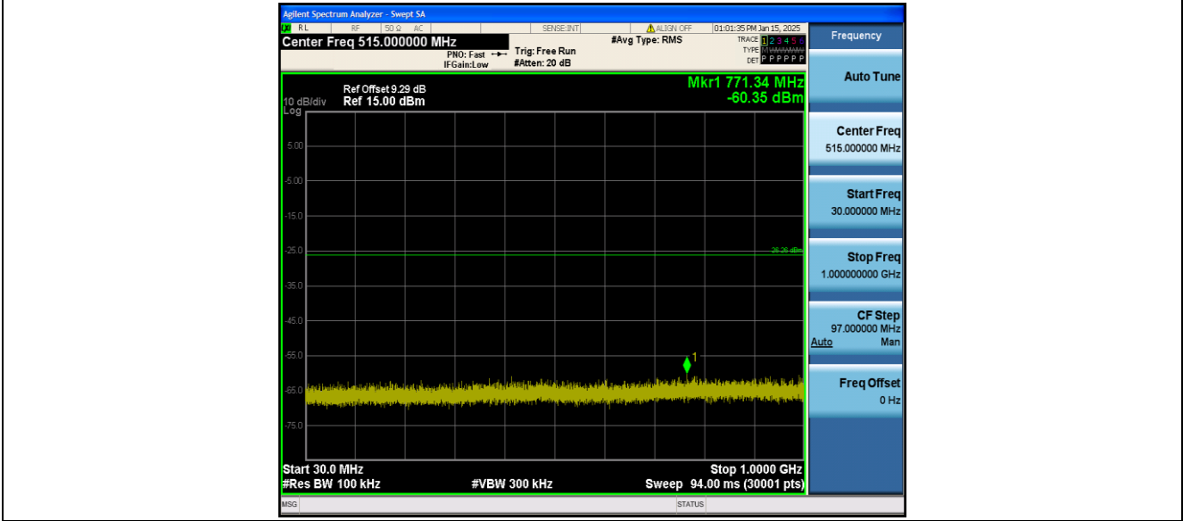
11B_Ant2_2412_30~1000
