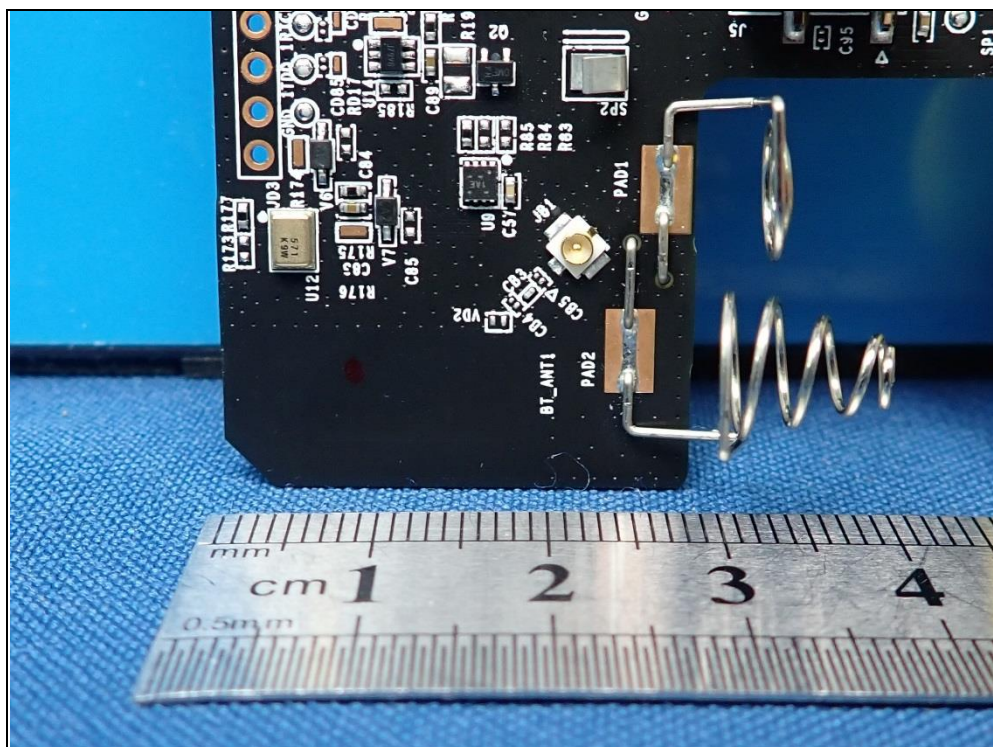
BLE antenna
