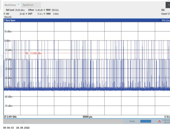
3DH1_Ant1_Hop
