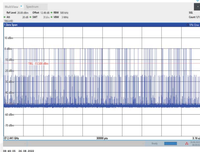
DH5_Ant1_Hop
