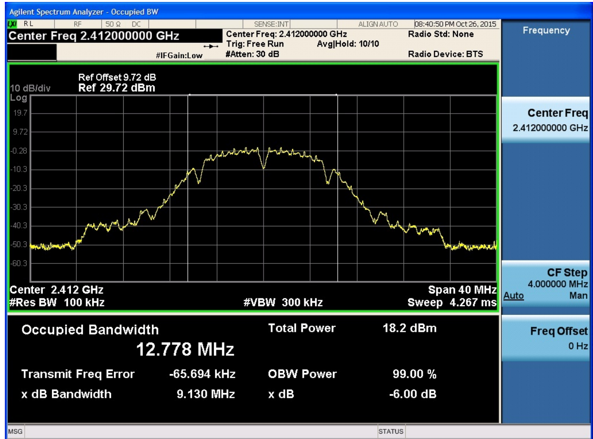
(Plot 4.7.1 A: Channel 1: 2412MHz @ 802.11b)
