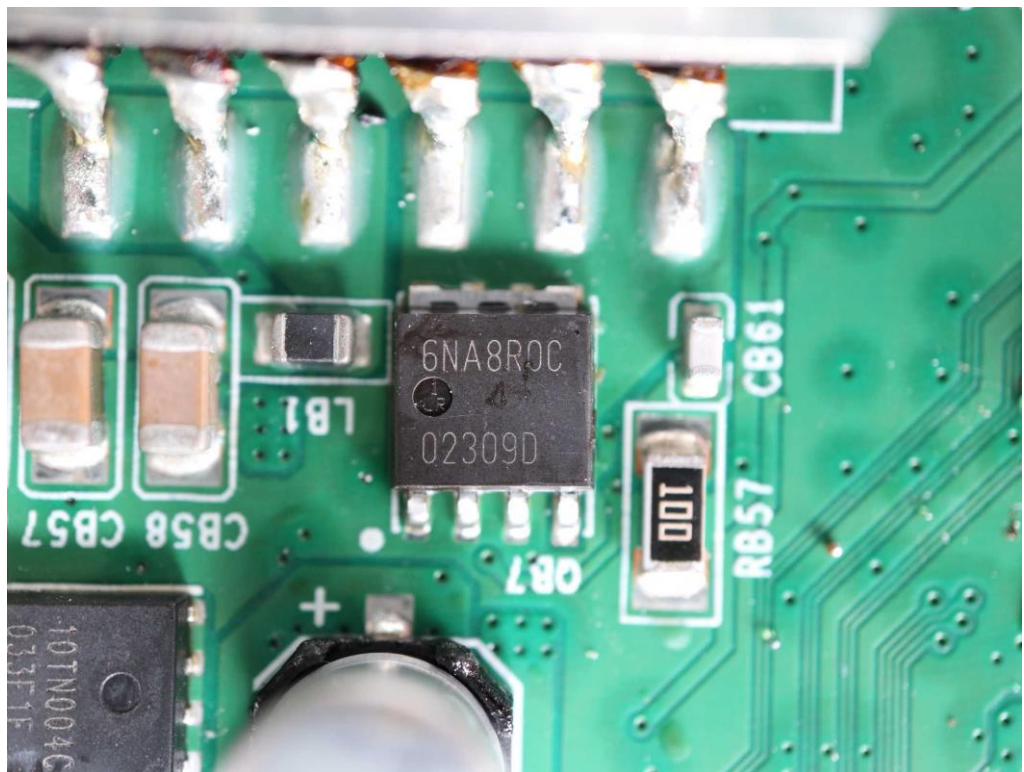
MOSFET (QB7) APEC / FET N 60V
