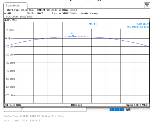
\pi/4 -DQPSK_High
