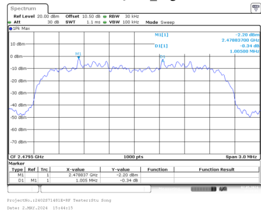
\pi/4 -DQPSK_High
