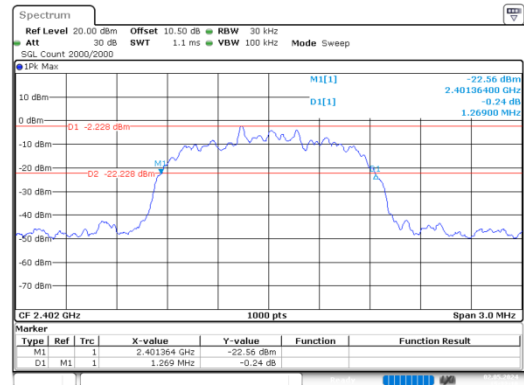
\pi/4 -DQPSK_Low
