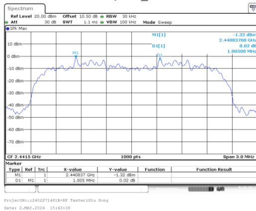
\pi/4 -DQPSK_Middle
