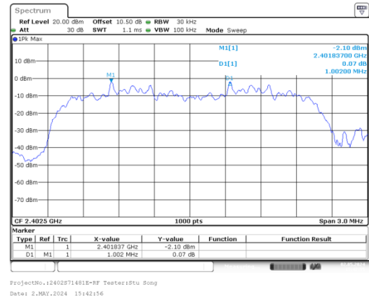
\pi/4 -DQPSK_Low
