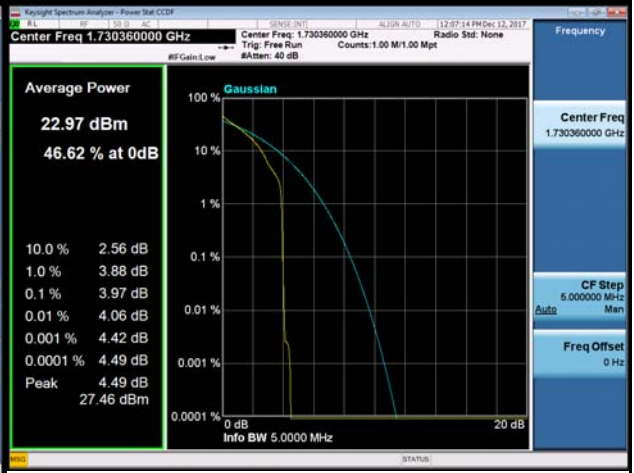
16QAM-19975
