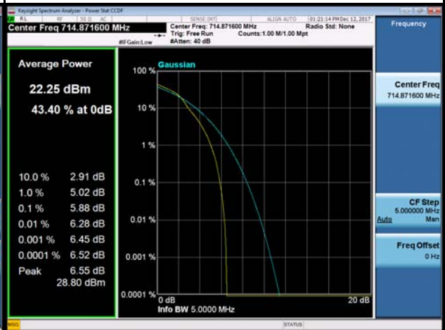
16QAM-23173
