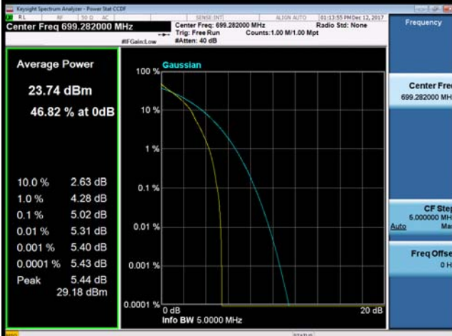
QPSK-23165
