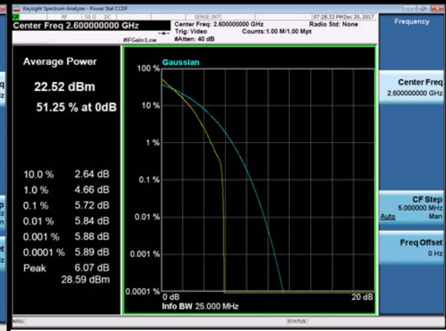
16QAM-40190
