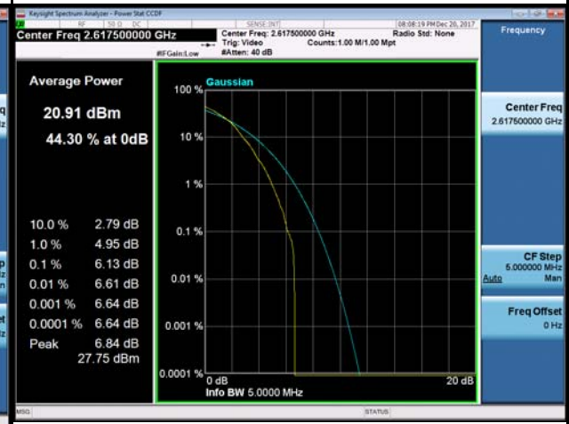
16QAM-38225
