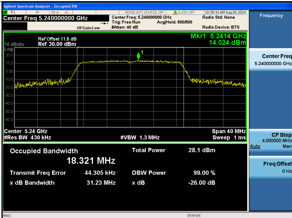
11N20MIMO-Ant3-5240
