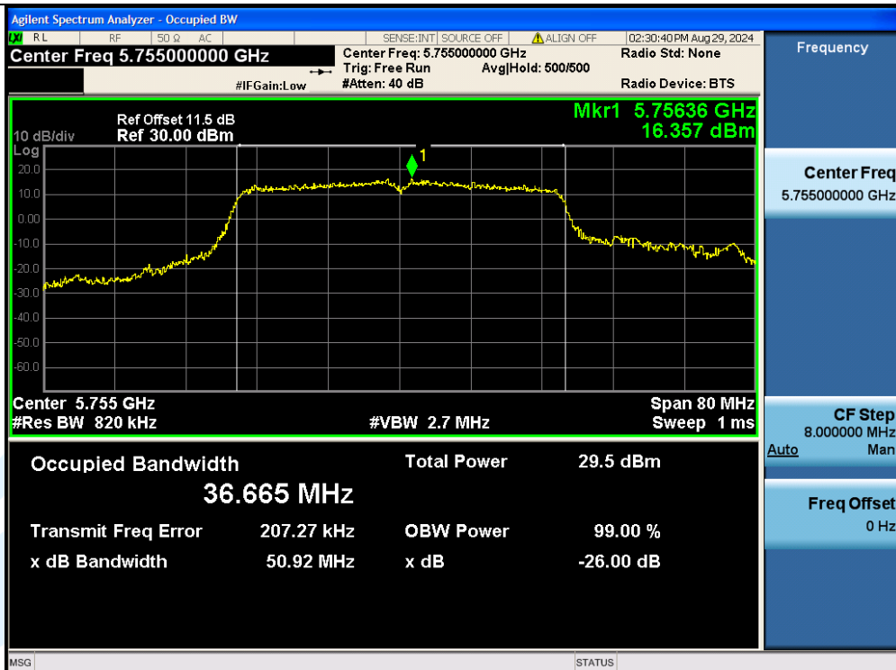
11N40MIMO-Ant3-5755
