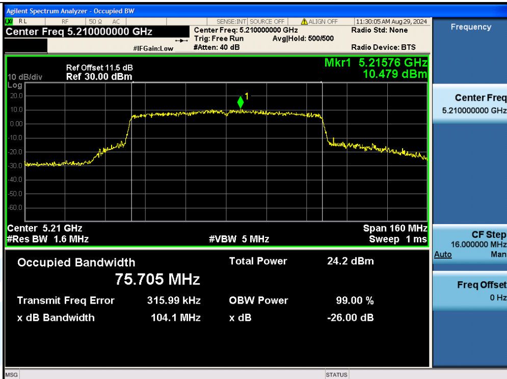
11AC80MIMO-Ant3-5210
