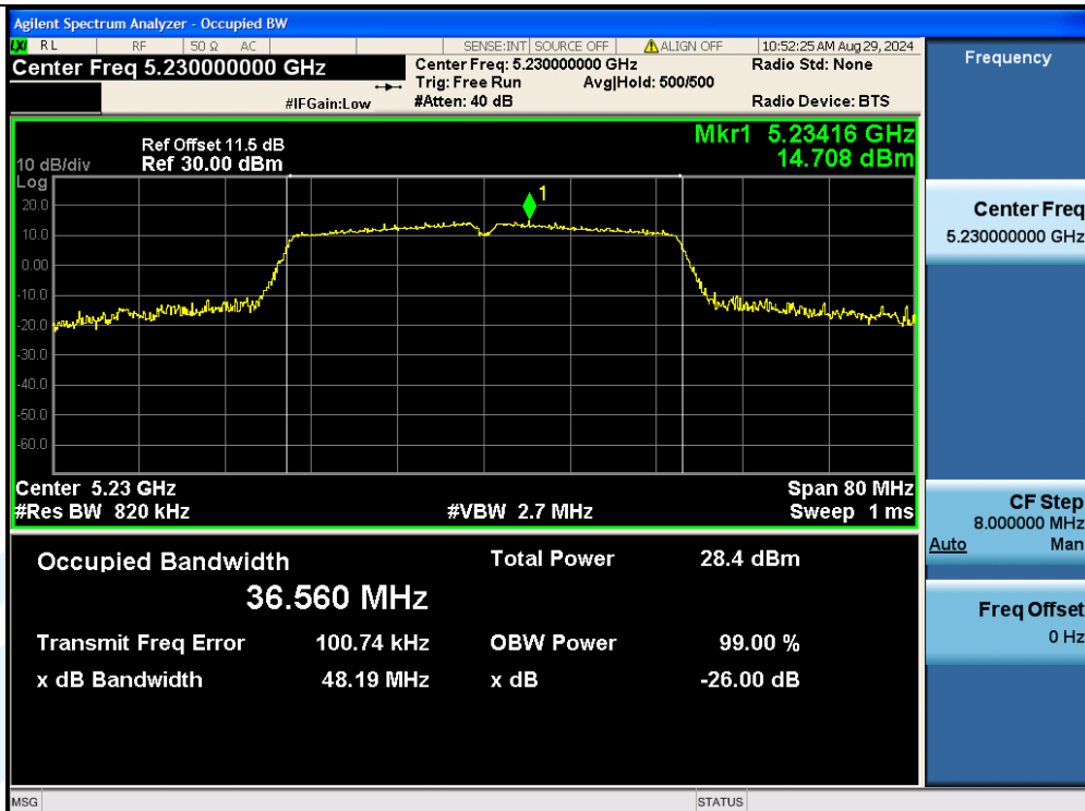
11N40MIMO-Ant3-5230
