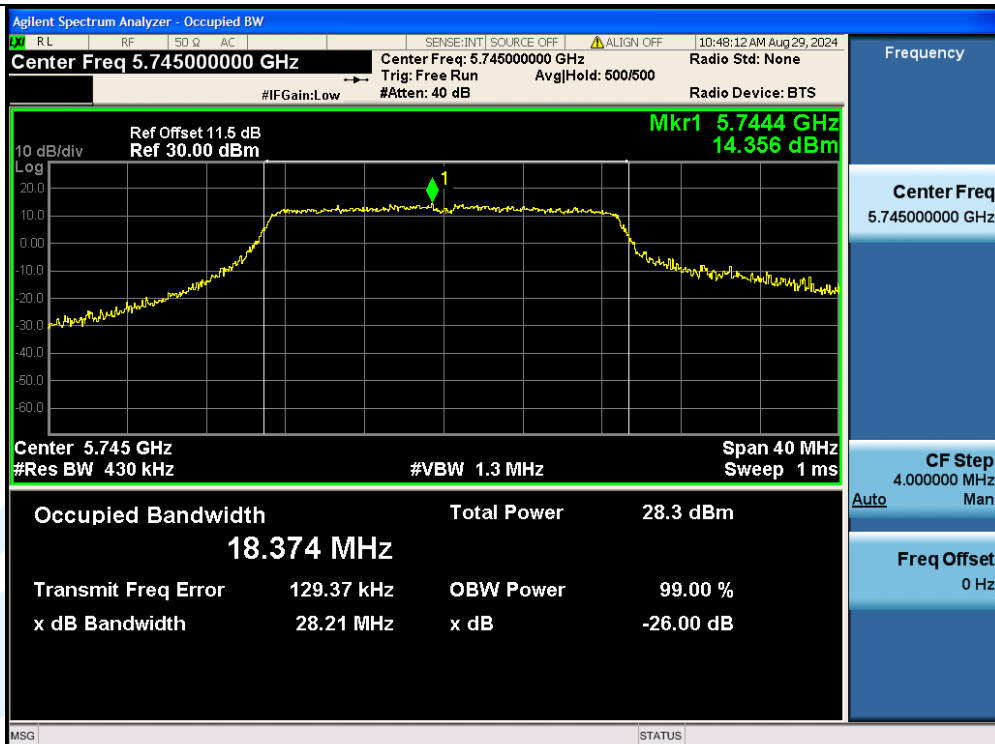
11N20MIMO-Ant3-5745
