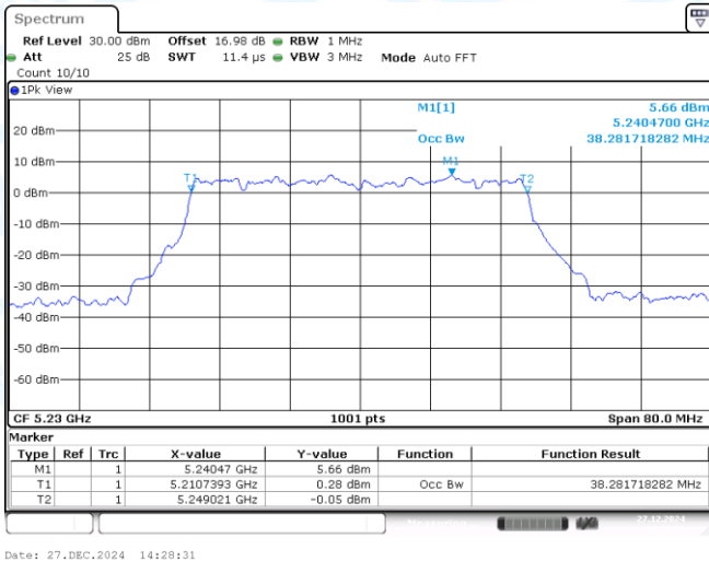
11AX40MIMO-Ant1-5230
