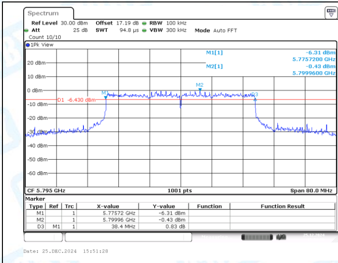
11AX40MIMO-Ant1-5795-PASS
