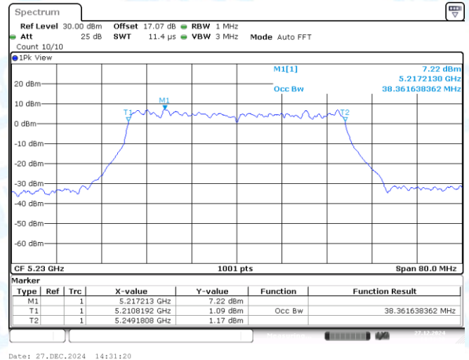
11AX40MIMO-Ant2-5230
