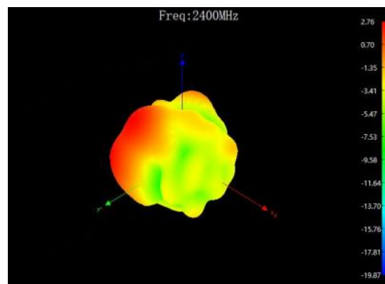
2400MHz 3D
