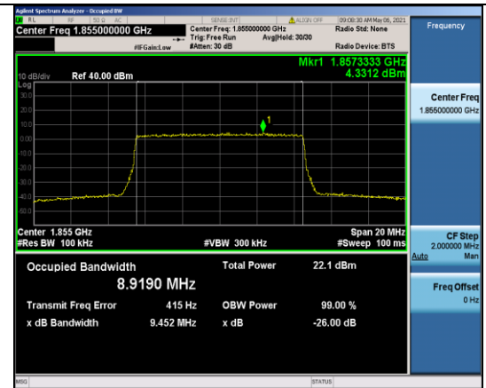
Band2-10MHz-16QAM-18650-50RB#0-8.9190
