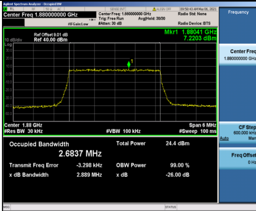
Band2-3MHz-QPSK-18900-15RB#0-2.6837
