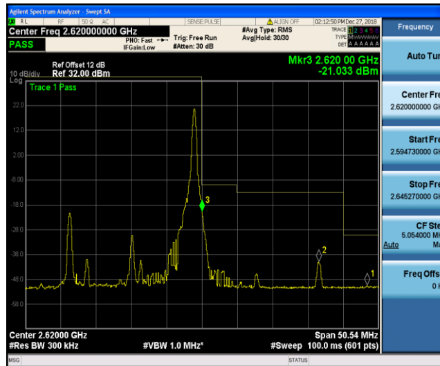
Band38_20MHz_QPSK_38150_1RB#99
