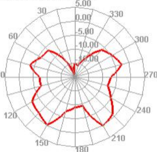
2450.000MHz E2
