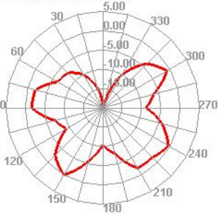
2450.000MHz E1
