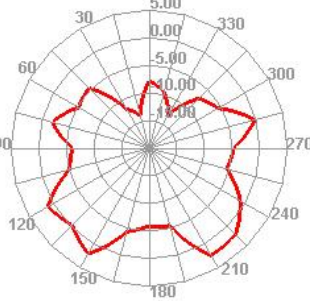
2500.000MHz E2
