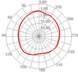
2450.000MHz H
