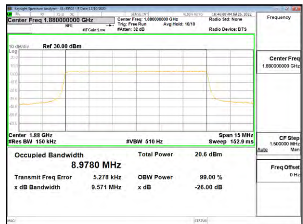
LTE2 10MHz QPSK MID Ch RB25-0
