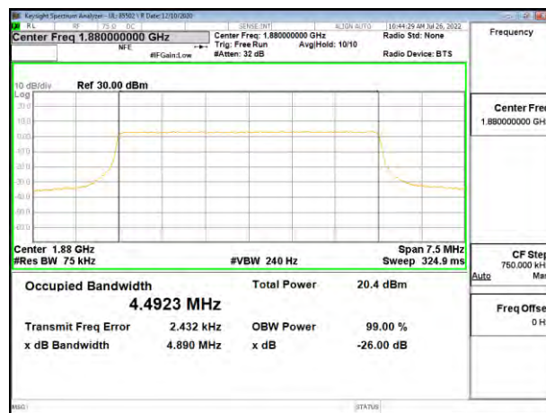
LTE2 5MHz QPSK MID Ch RB50-0
