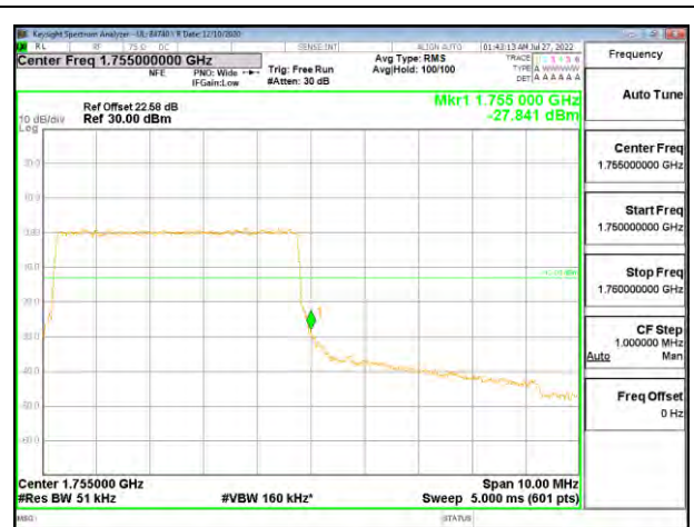
LTE 5MHz QPSK HIGH Ch RB25-0
