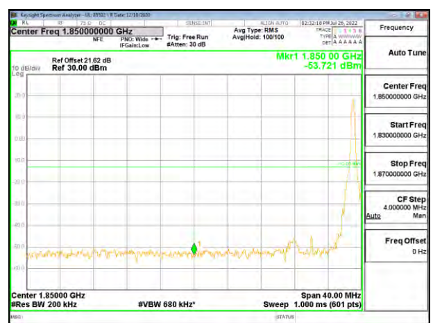
LTE2 20MHz 16QAM LOW Ch RB1-99
