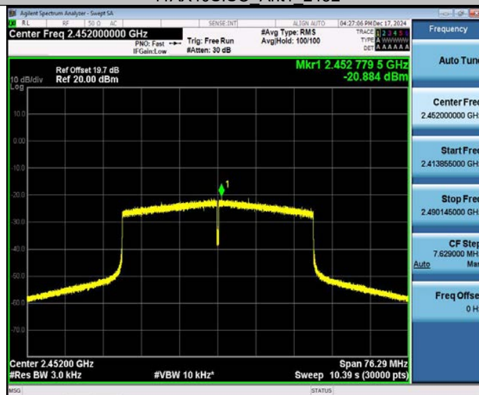
11AX40SISO_Ant1_2452
