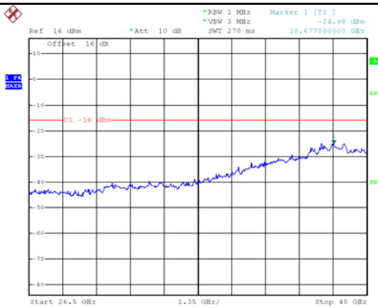
10MHz - Low CH 26.5GHz~40GHz
