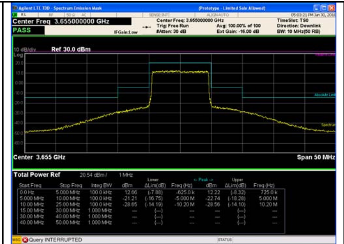
10MHz - Low CH 64QAM
