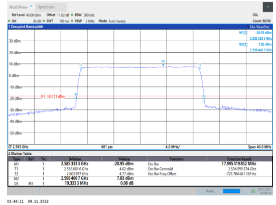
Band41-20MHz-QPSK-40640-100RB#0
