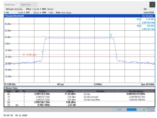
Band41-10MHz-QPSK-40640-50RB#0
