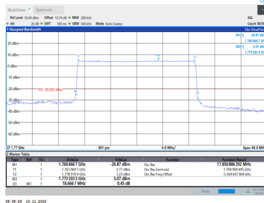
Band66-20MHz-QPSK-132572-100RB#0
