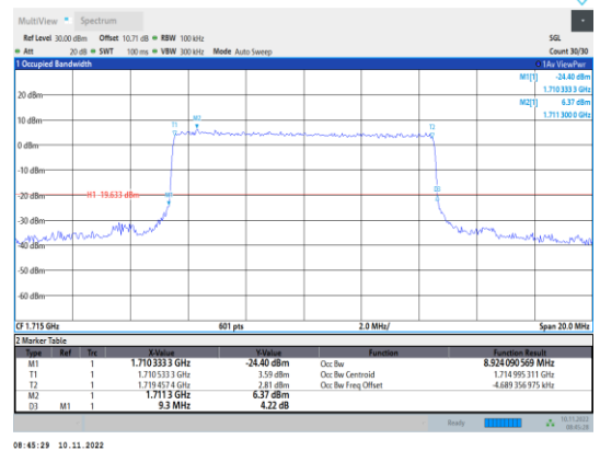
Band66-10MHz-QPSK-132022-50RB#0
