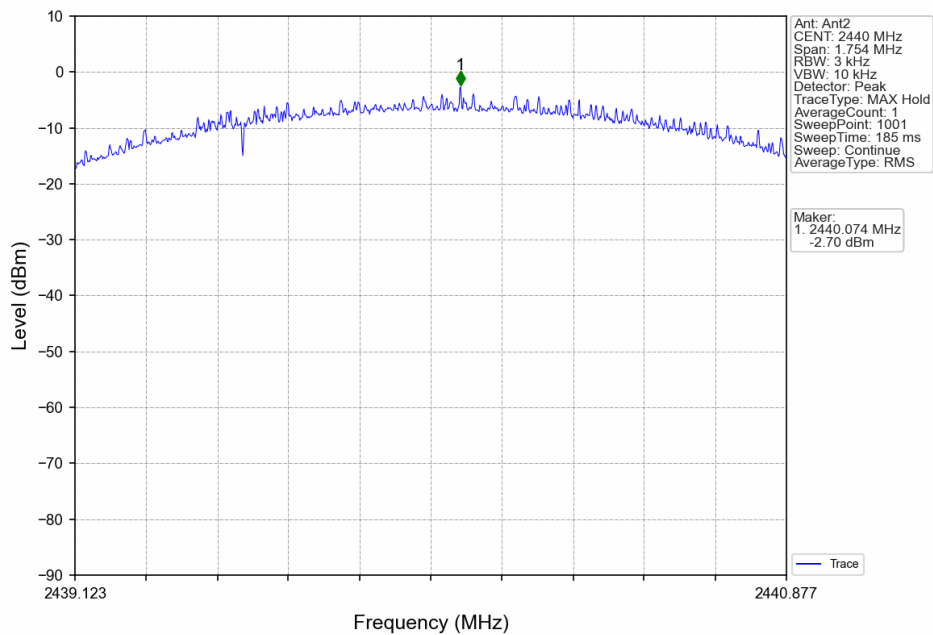
2M_MCH_2440MHz_Ant2_NTNV
