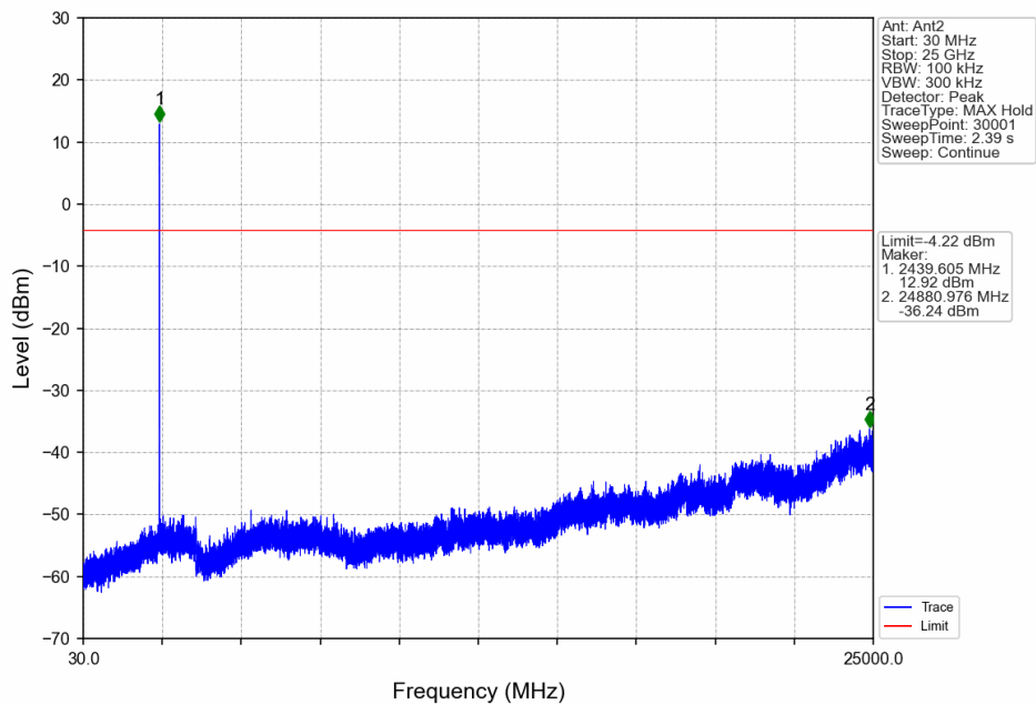
1M_MCH_2440MHz_Ant2_NTNV
