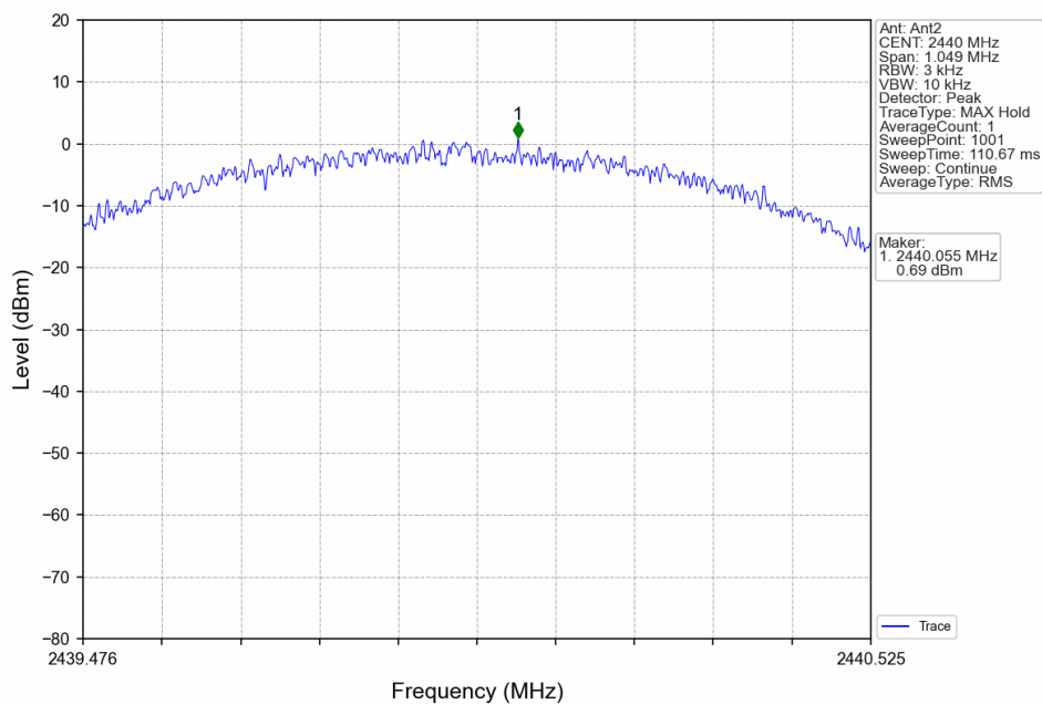
1M_MCH_2440MHz_Ant2_NTNV
