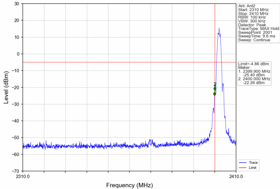
2M_LCH_2402MHz_Ant2_NTNV
