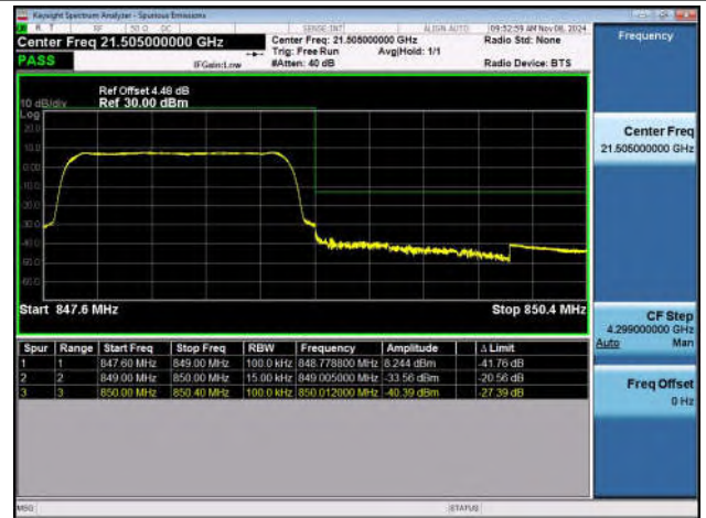
Band5_3MHz_QPSK_20635_15RB#0
