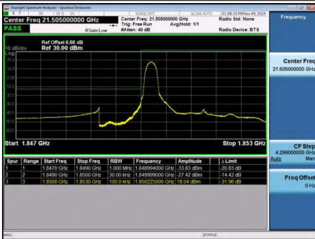
Band2_3MHz_QPSK_18615_1RB#0
