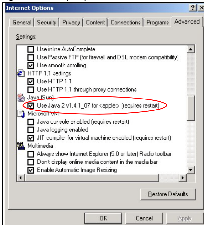
Figure 125 Java (Sun)
