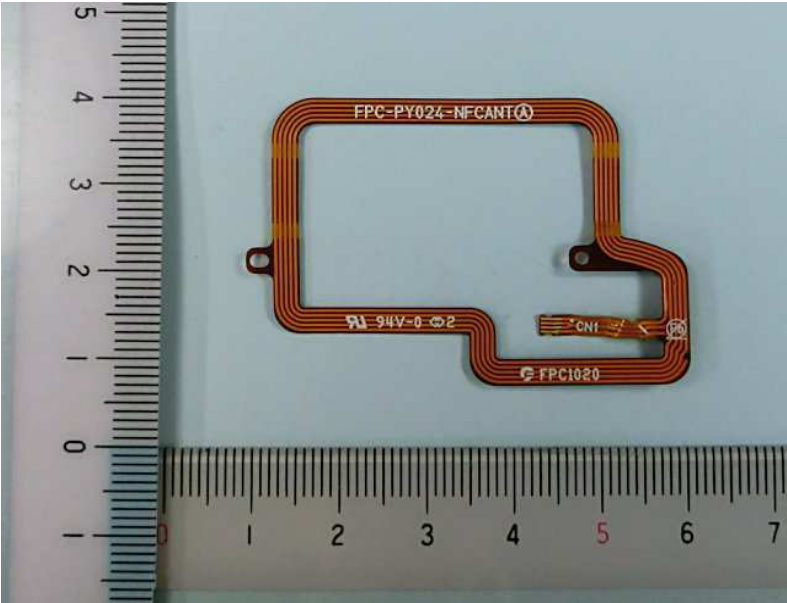
NFC Antenna
