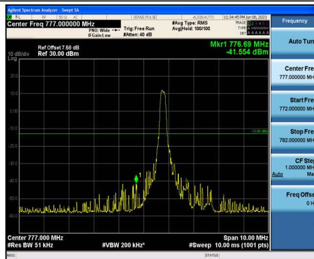
Band13-10MHz-QPSK-23230-1-0-Low--41.55-PASS
