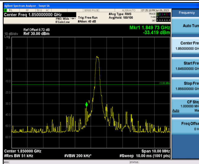
Band2-3MHz-QPSK-18615-1-0-Low--33.42-PASS
