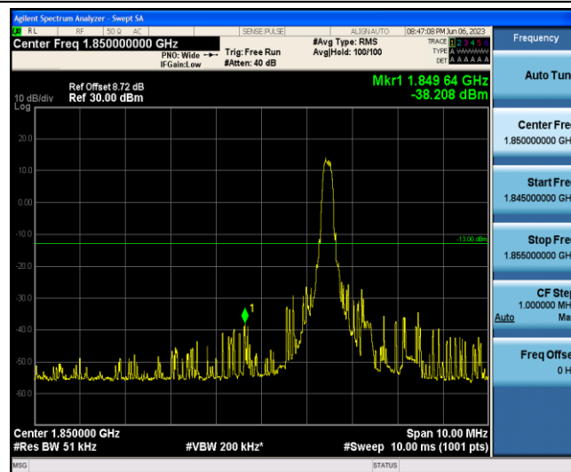
Band2-20MHz-QPSK-18700-1-0-Low--38.21-PASS
