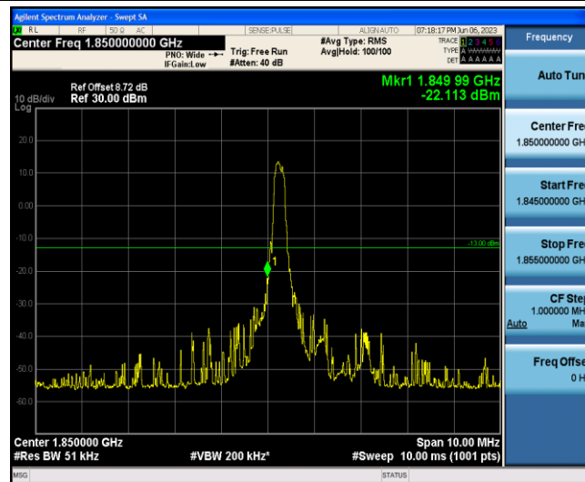
Band2-1.4MHz-QPSK-18607-1-0-Low--22.11-PASS
