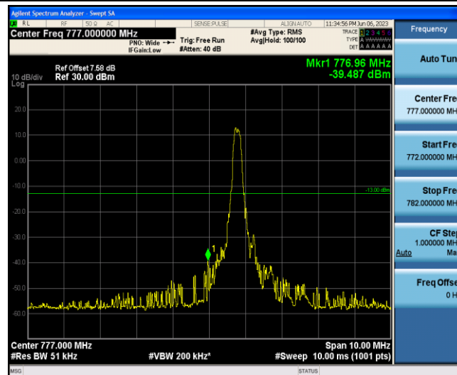
Band13-10MHz-16QAM-23230-1-0-Low--39.49-PASS
