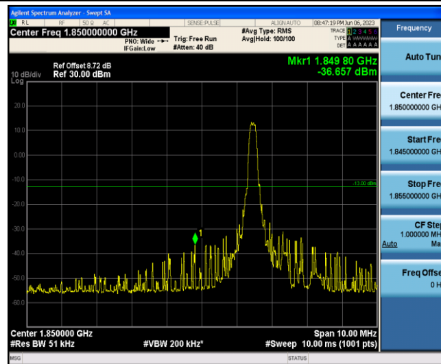
Band2-20MHz-16QAM-18700-1-0-Low--36.66-PASS
