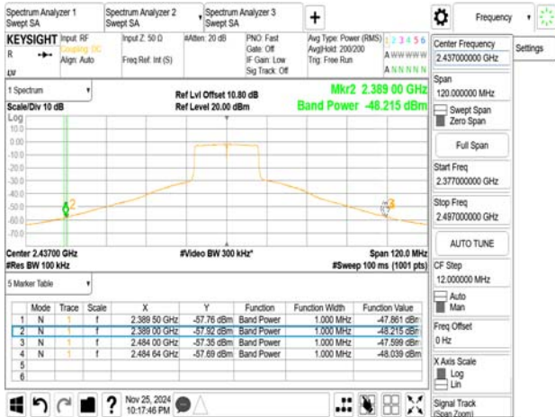
802.11ax_20MHz_2437MHz_RU26_0
