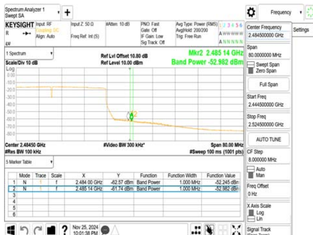
802.11ax_40MHz_2462MHz
