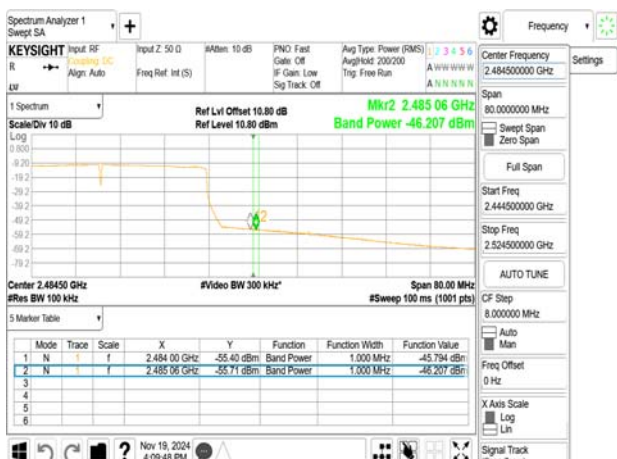
802.11ax_40MHz_2457MHz
