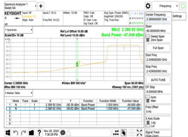
802.11ax_20MHz_2417MHz_RU26_0
