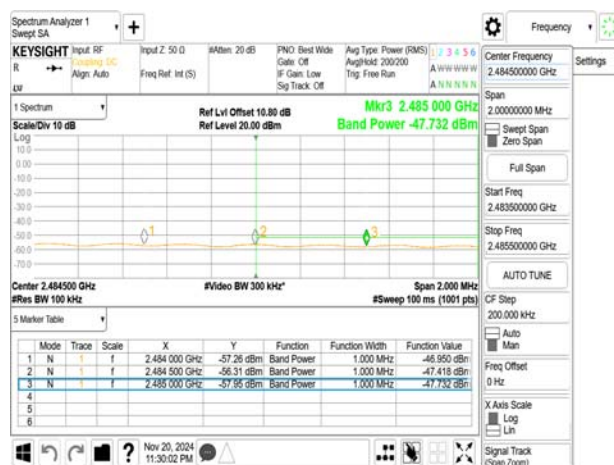
802.11n_20MHz_2457MHz
