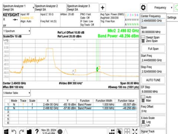
802.11ax_20MHz_2462MHz_RU52_40
