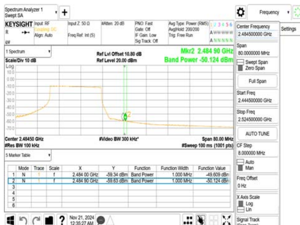
802.11ax_40MHz_2457MHz_RU484
