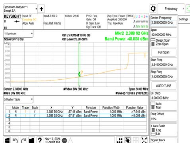
802.11ax_20MHz_2427MHz
