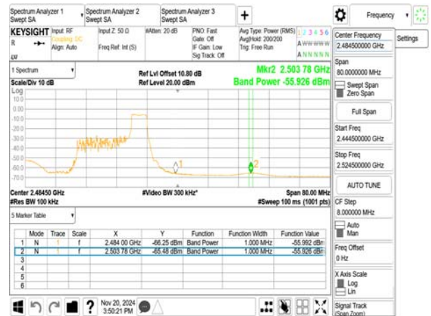
802.11ax_20MHz_2472MHz
