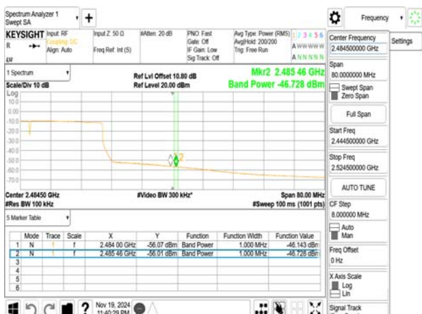
802.11ax_40MHz_2447MHz
