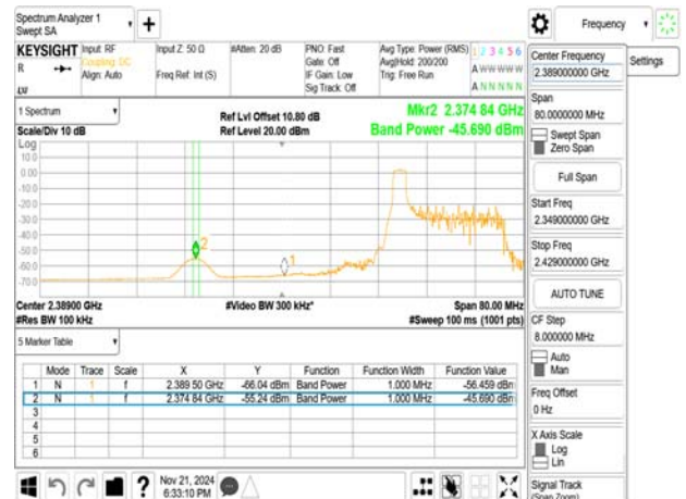
802.11ax_20MHz_2417MHz_RU52_37
