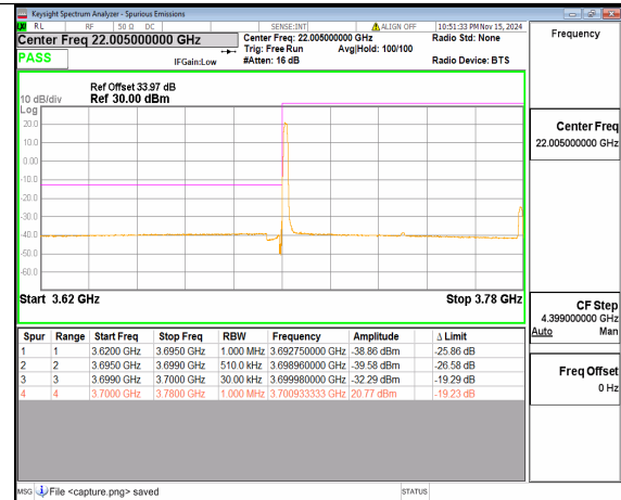
n77(3700-3980MHz) 80M DFT-s-OFDM QPSK Edge 1RB Left Low
