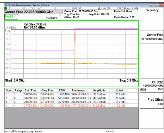
n77(3700-3980MHz) 100M DFT-s-OFDM BPSK Edge 1RB Left Low
