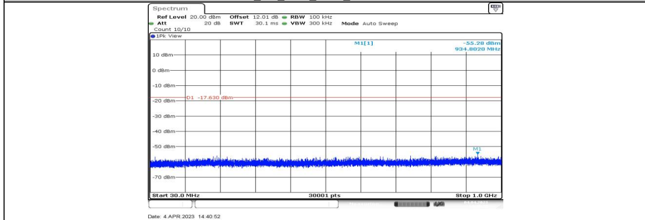
BLE_2M_Ant1_2480_30~1000
