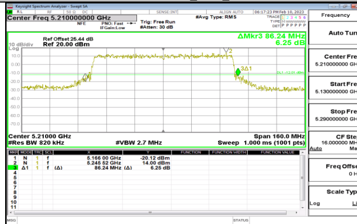
11AX80MIMO_Ant1_5210
