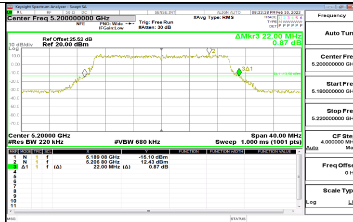
11BE20MIMO_Ant3_5200
