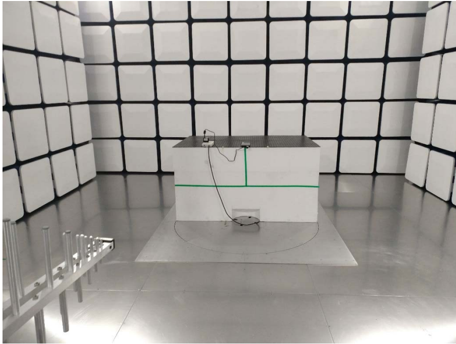
Blow 1GHz-BT/BLE/WIFI
