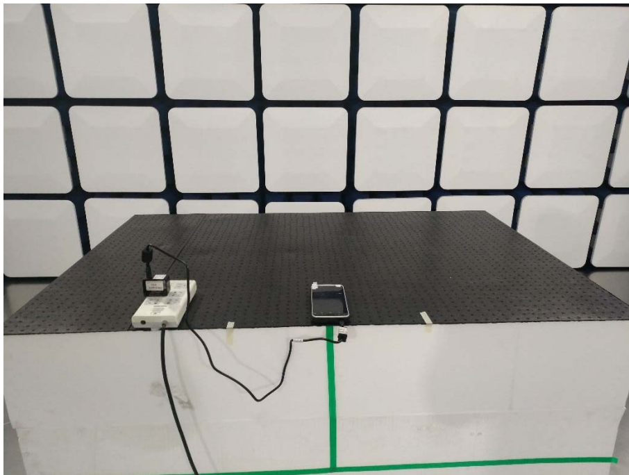
Close-up-BT/BLE/WIFI
