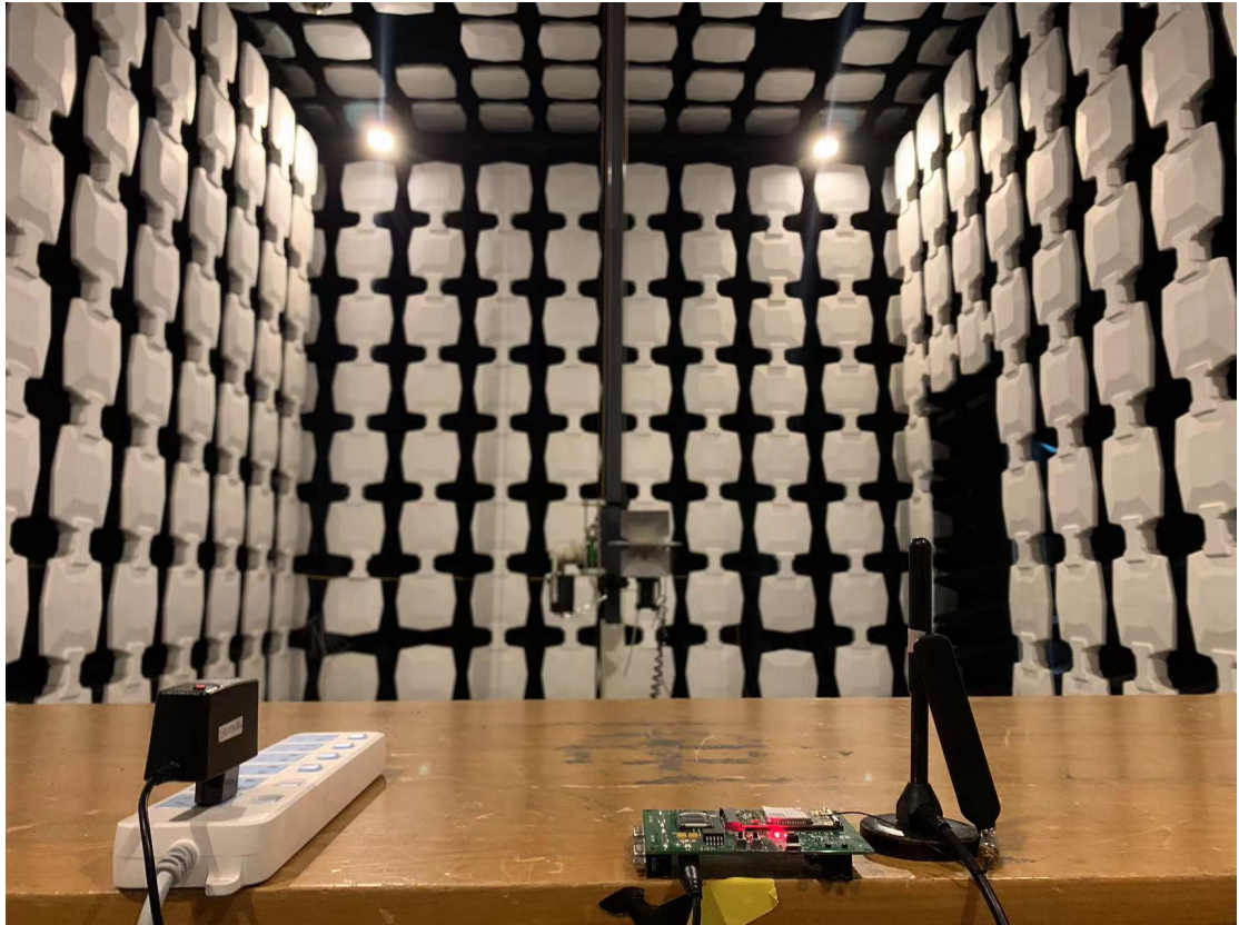
A7672SA miniPCIE RE 1GHz-18GHz
