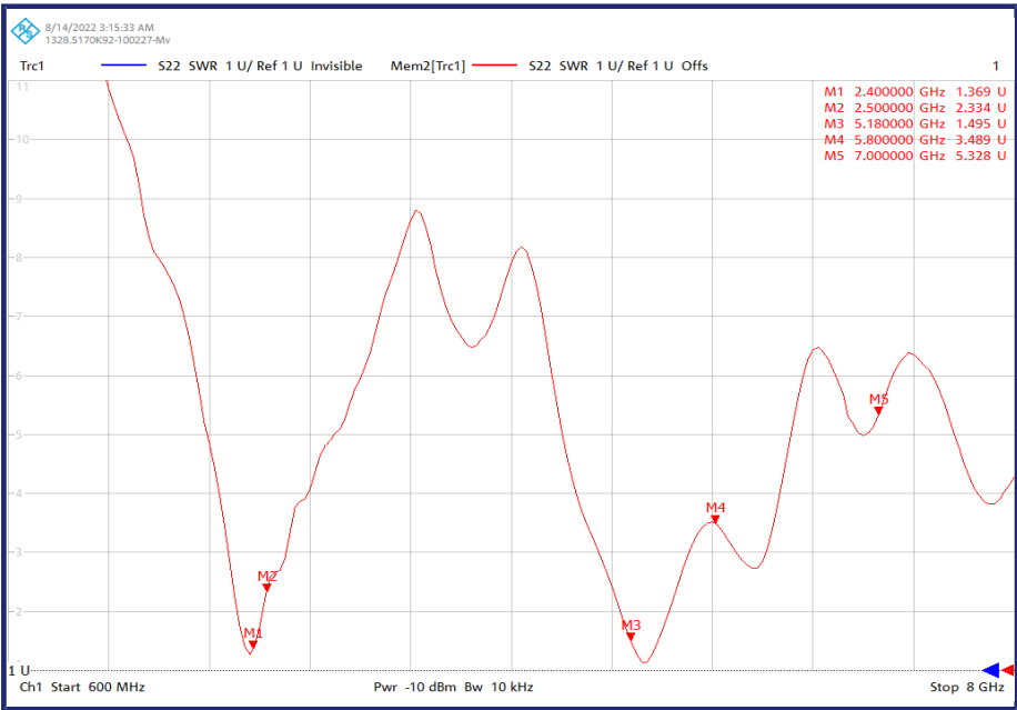
ANT2天线
