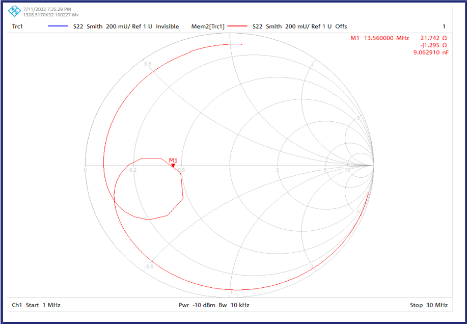
NFC天线
