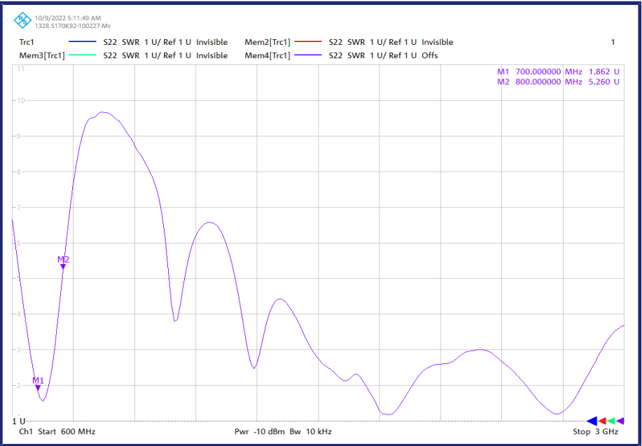
ANT0/RF4天线
