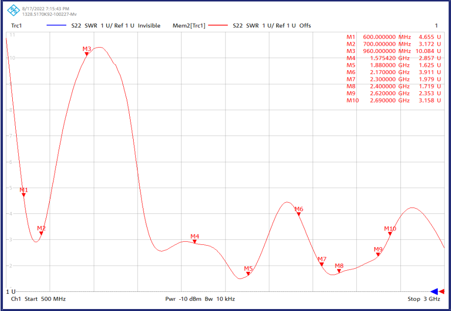
ANT5天线
