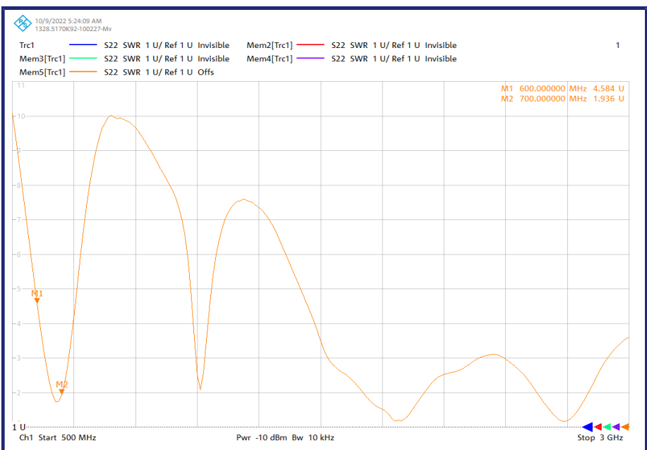
ANT0/RF4天线
