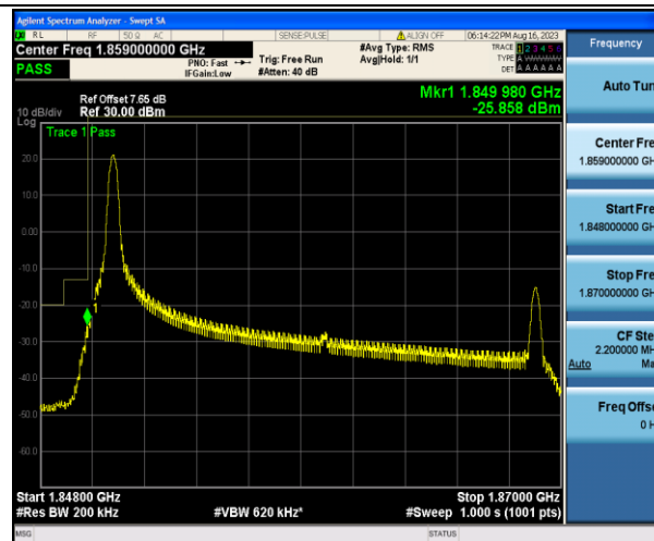
Band2_20MHz_QPSK_18700_1RB#0
