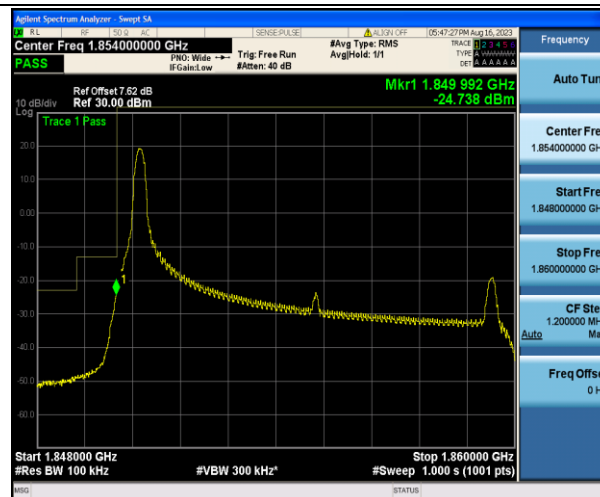
Band2_10MHz_QPSK_18650_1RB#0
