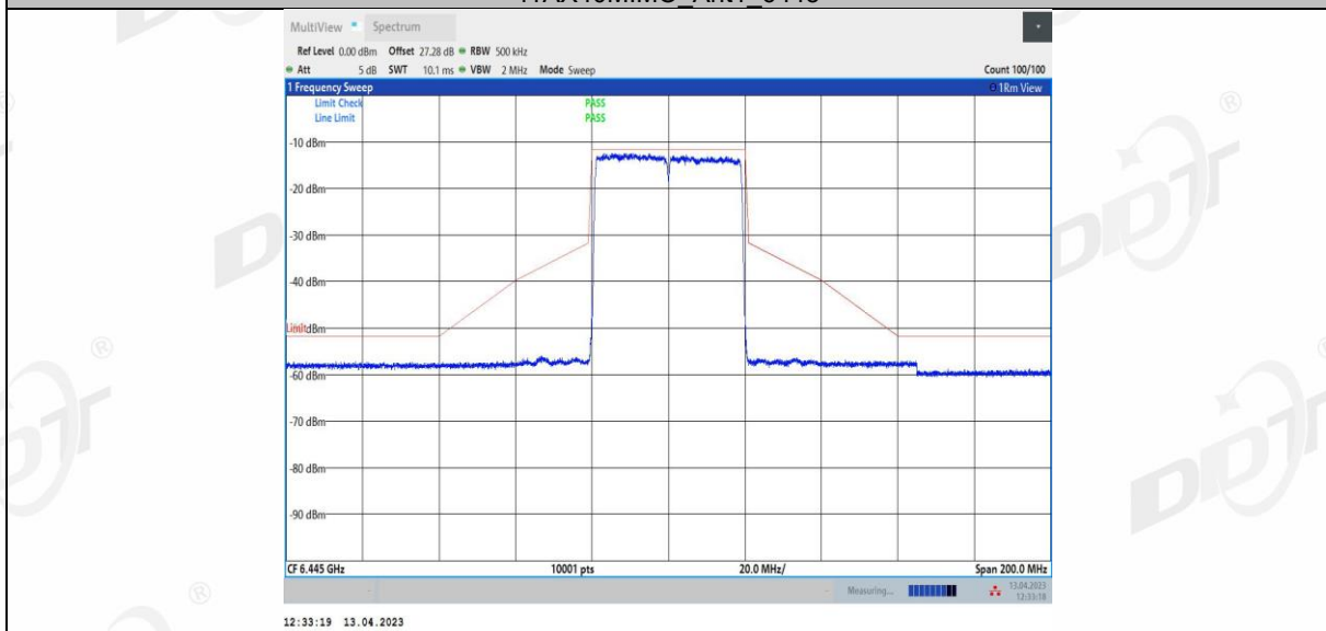
11AX40MIMO_Ant2_6445
