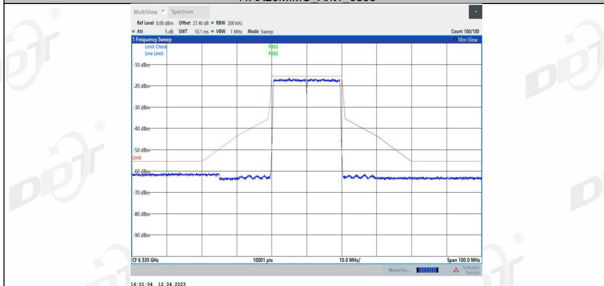
11AX20MIMO_Ant2_6535
