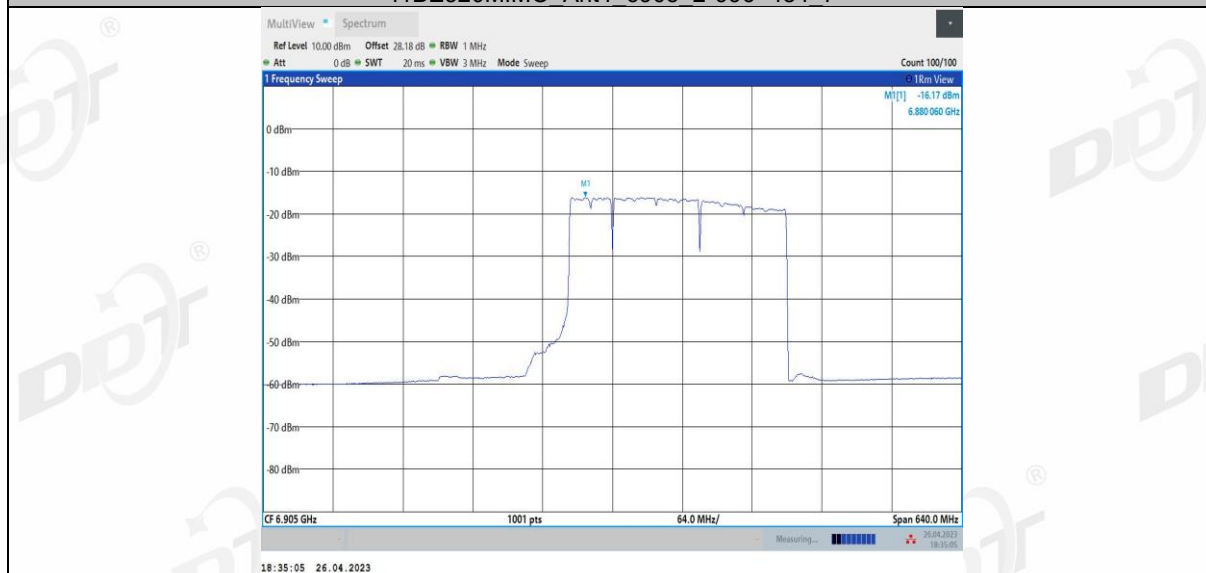
11BE320MIMO Ant4 6905 2*996+484 8
