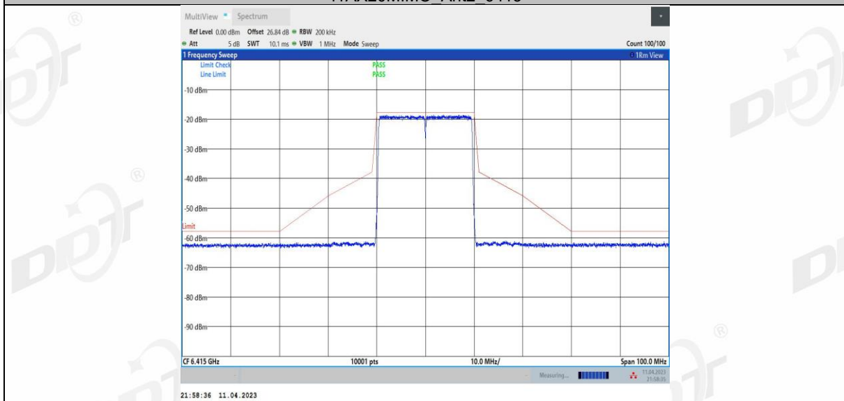
11AX20MIMO_Ant3_6415
