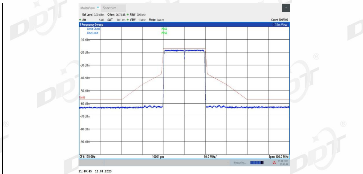
11AX20MIMO_Ant3_6175
