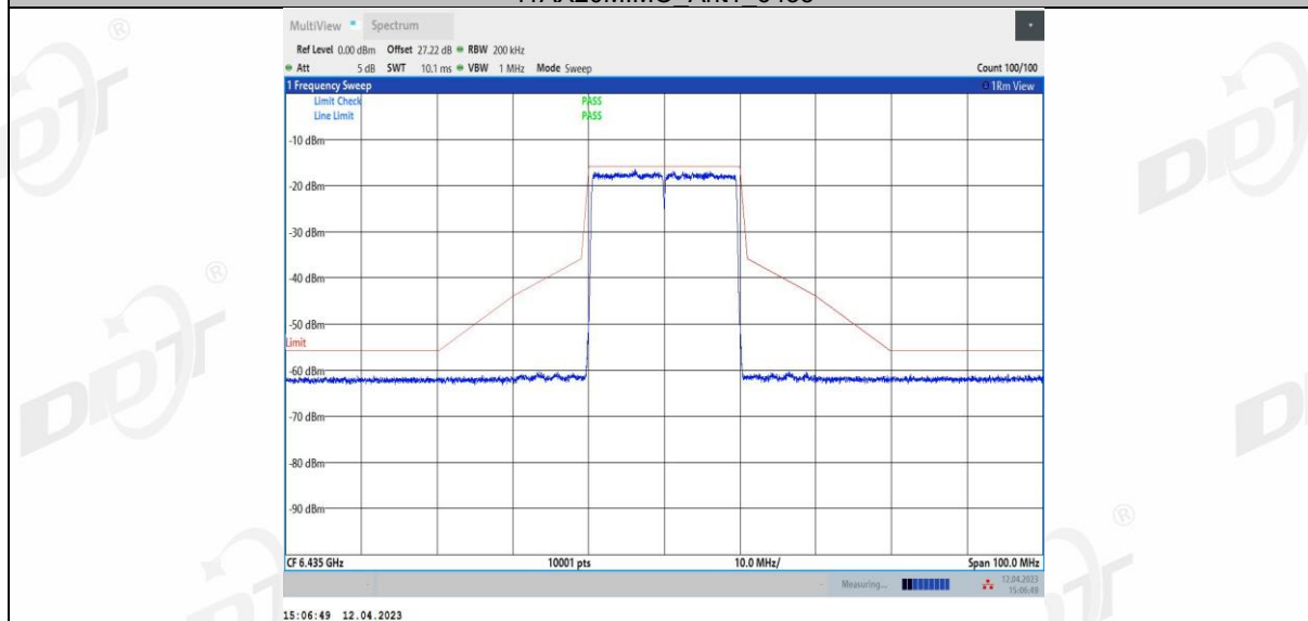
11AX20MIMO_Ant2_6435
