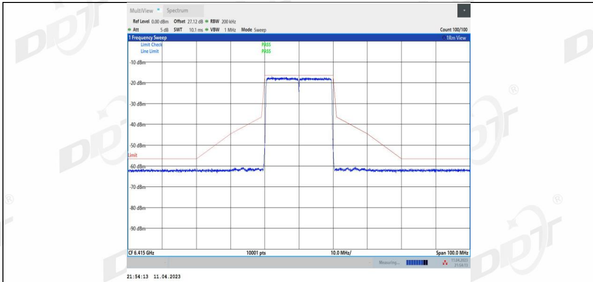
11AX20MIMO_Ant2_6415
