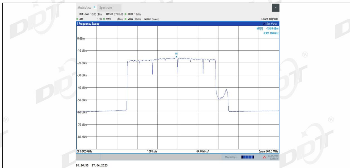
11BE320MIMO Ant4 6905 2*996+484 7
