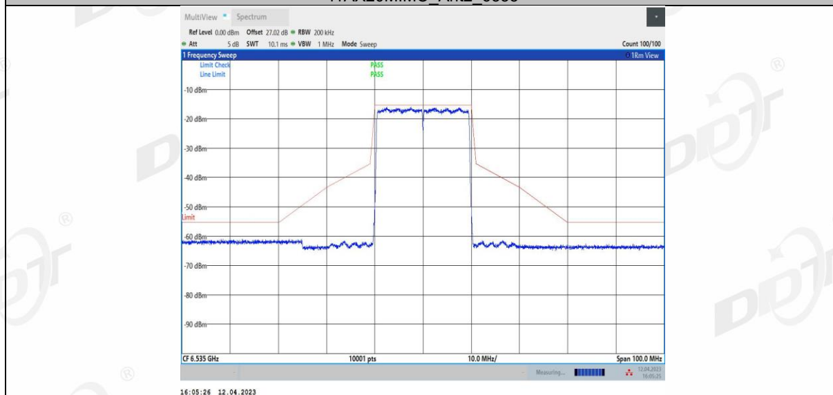
11AX20MIMO_Ant3_6535
