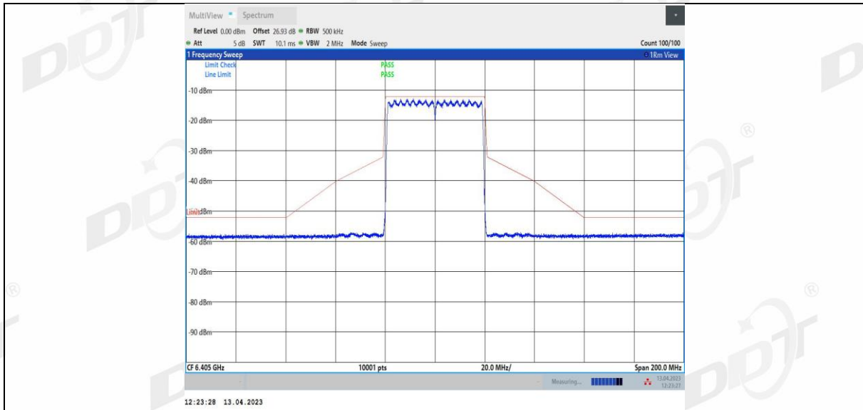
11AX40MIMO_Ant4_6405
