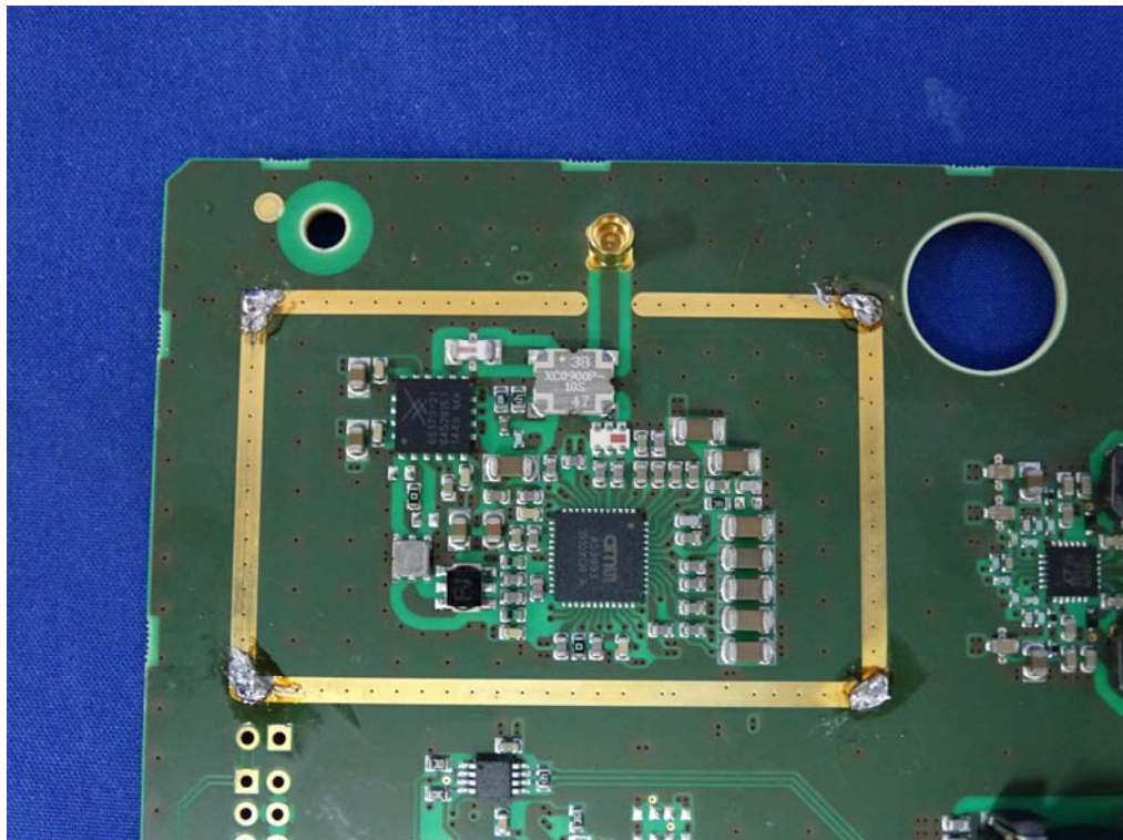
(9) EUT Photo-RF Module
