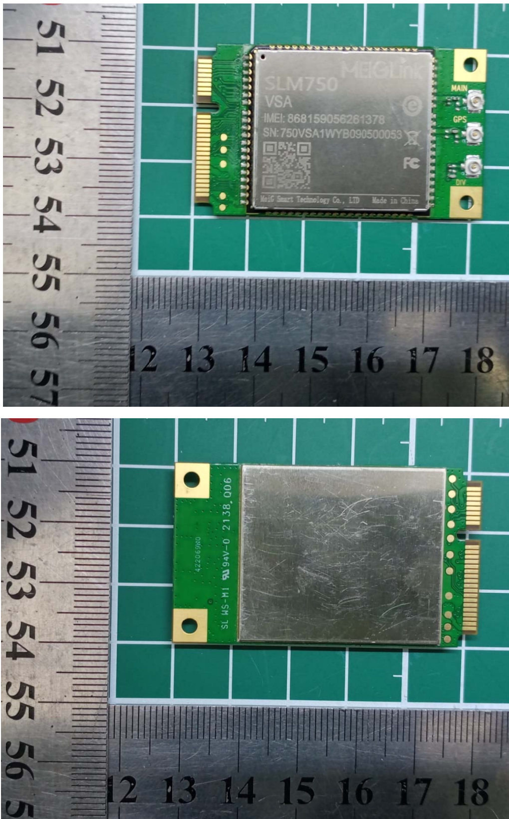
a: EUT
