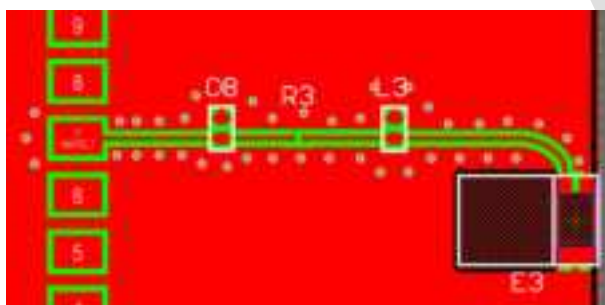
BLE Layout
