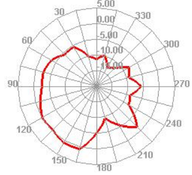
2500.000MHz E1
