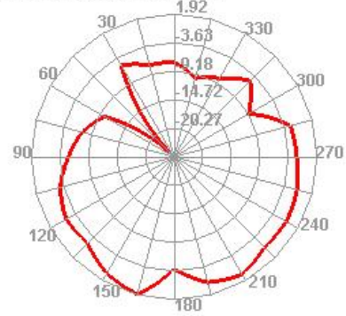
2450.000MHz E2
