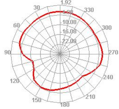
2450.000MHz H
