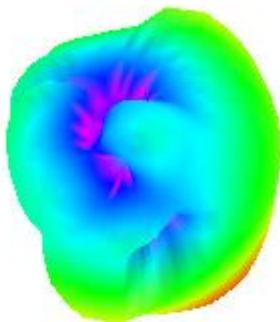
2400.000MHz
