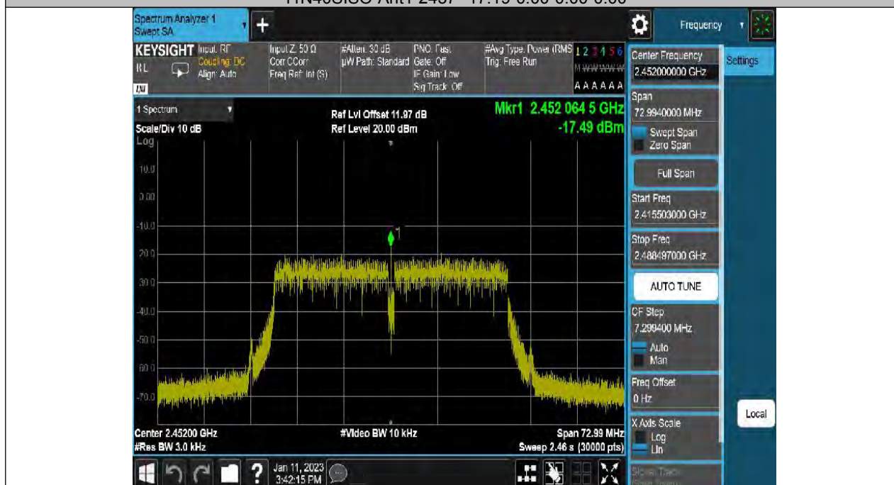
11N40SISO-Ant1-2452--17.49-0.00-0.00-0.00
