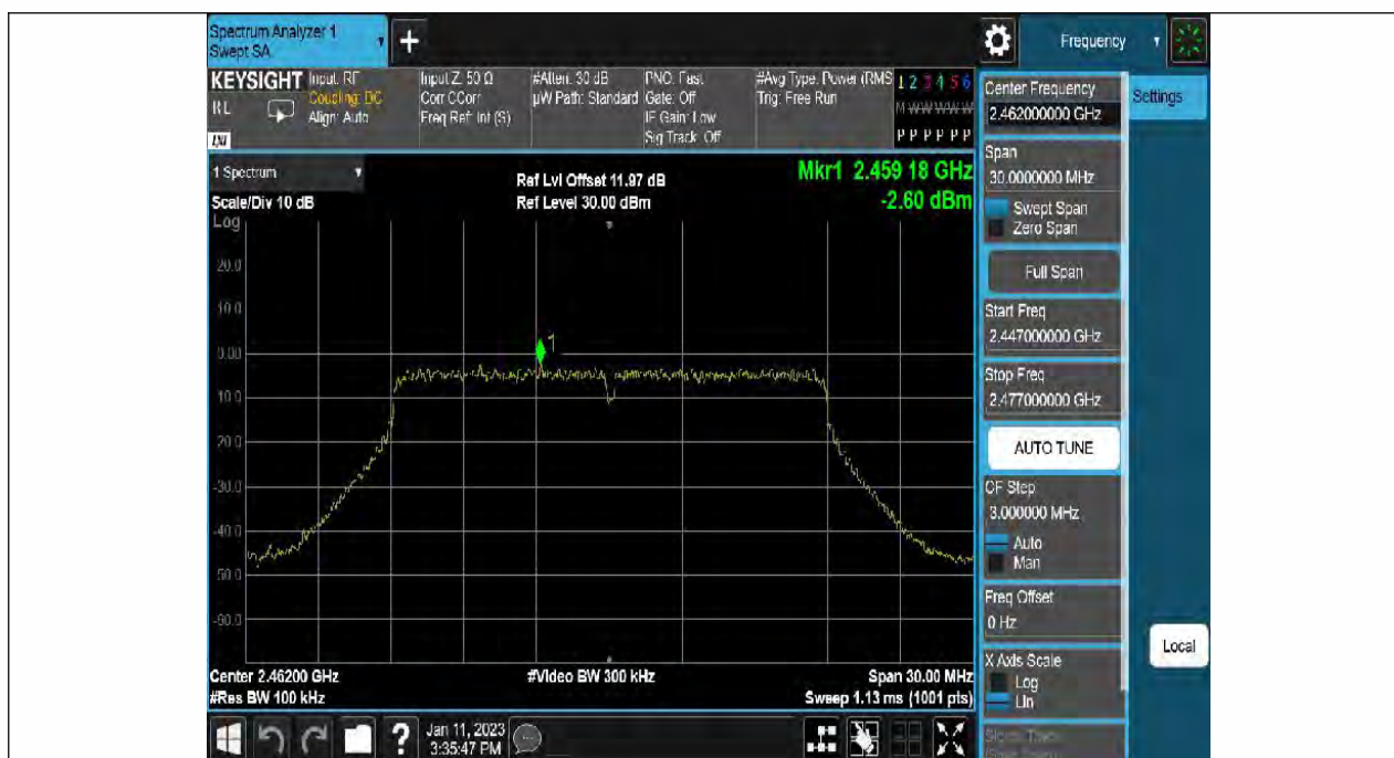
11N20SISO-Ant1-2462-0~Reference--2.60
