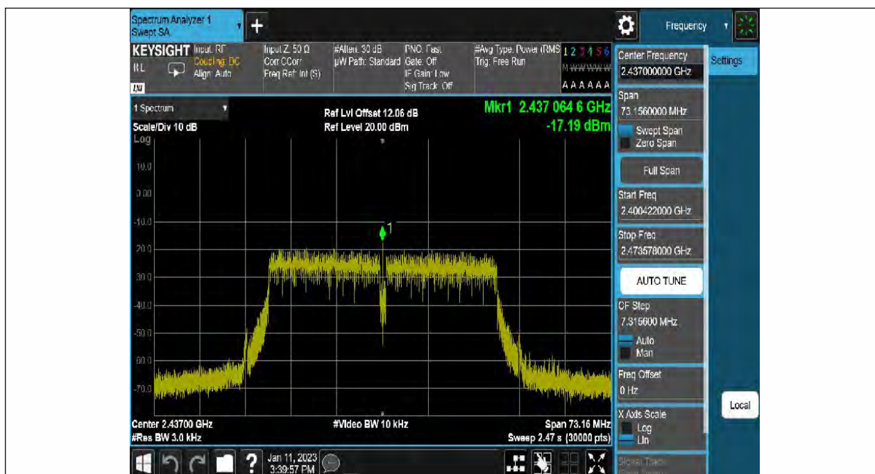
11N40SISO-Ant1-2437--17.19-0.00-0.00-0.00
