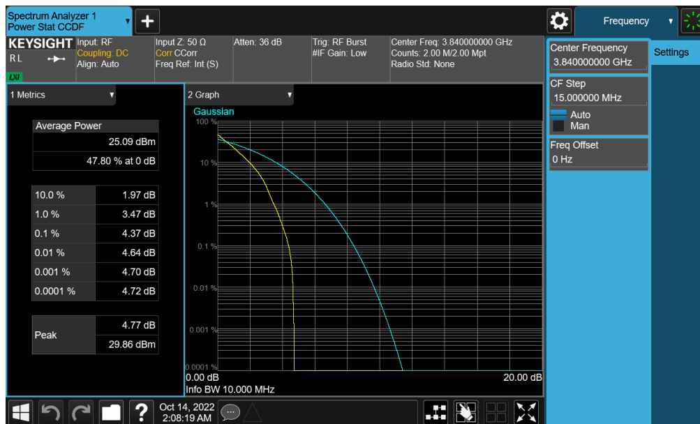
Plot 7-250. PAR Plot (NR Band n77 - C-Band – 10MHz DFT-s-OFDM \pi/2 BPSK - Full RB)
