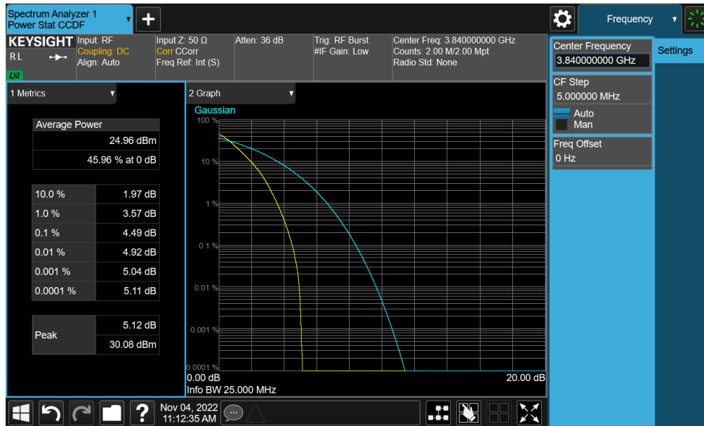
Plot 7-241. PAR Plot (NR Band n77 - C-Band – 25MHz DFT-s-OFDM \pi/2 BPSK - Full RB)
