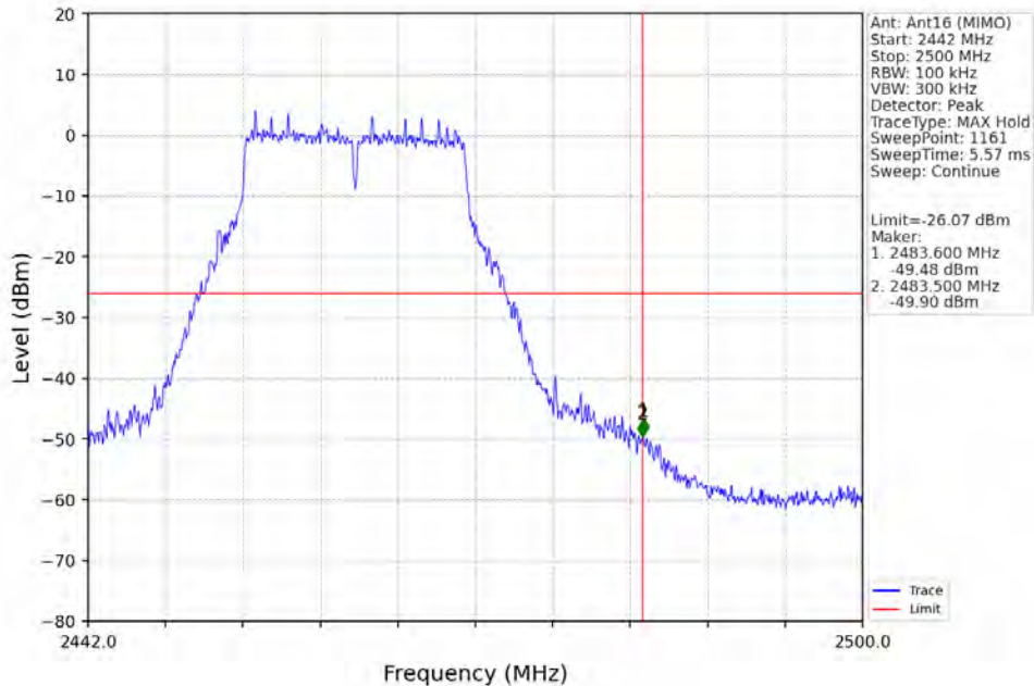
802.11g_HCH_2462MHz_Ant16 (MIMO)_NTNV
