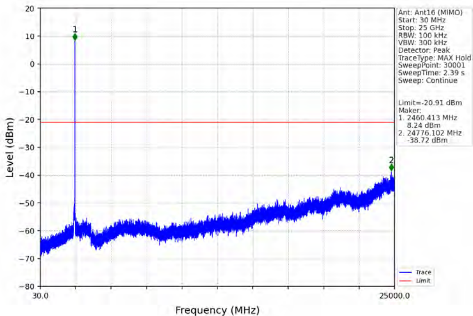
802.11b_HCH_2462MHz_Ant16 (MIMO)_NTNV
