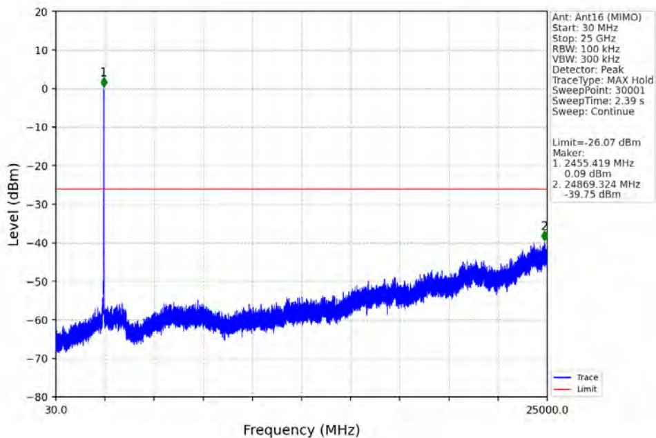
802.11g_HCH_2462MHz_Ant16 (MIMO)_NTNV
