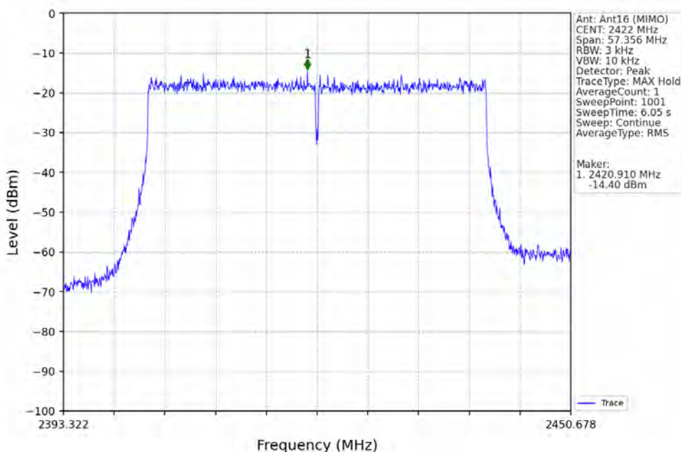
802.11ax(HEW40)_LCH_2422MHz_RU484_Left_Ant16 (MIMO)_NTNV
