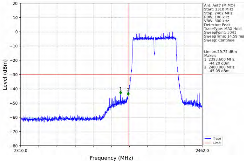
802.11n(HT40)_LCH_2422MHz_Ant7 (MIMO)_NTNV
