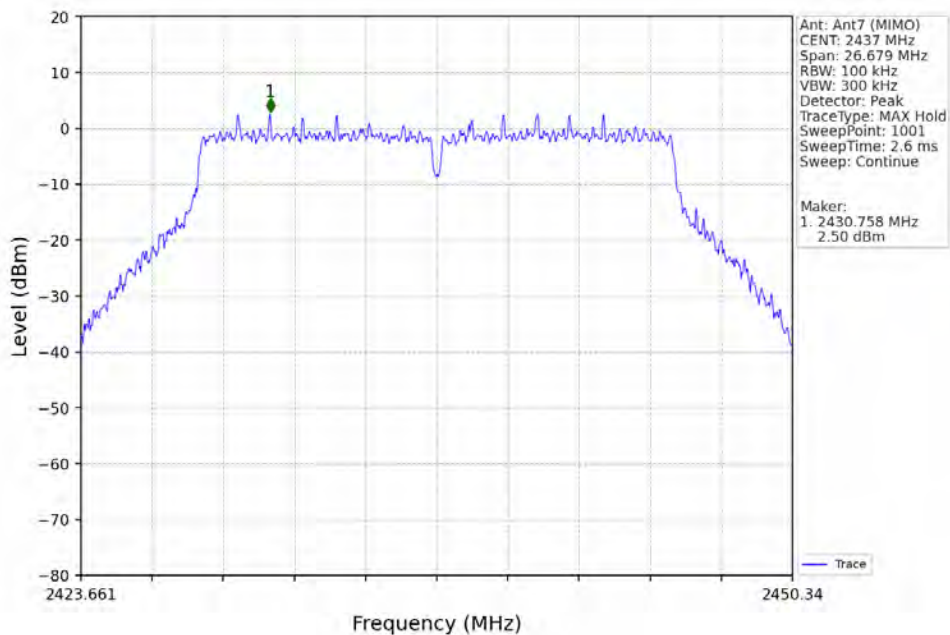
802.11n(HT20)_MCH_2437MHz_Ant7 (MIMO)_NTNV
