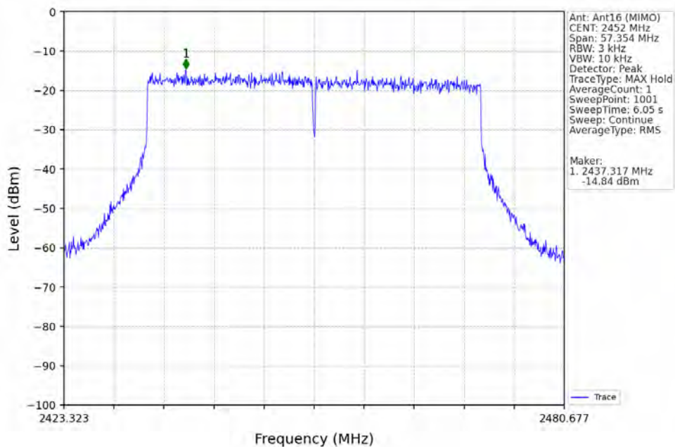
802.11be(EHT40)_HCH_2452MHz_RU484_Left_Ant16 (MIMO)_NTNV
