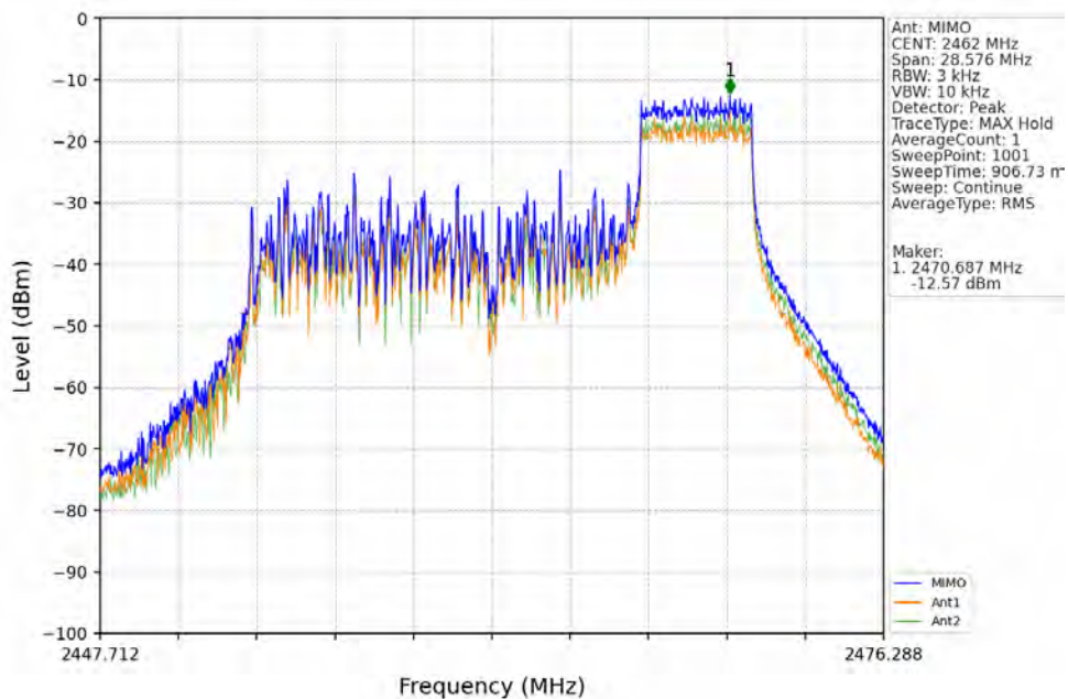
802.11be(EHT20)_HCH_2462MHz_RU52_Right_MIMO_NTNV
