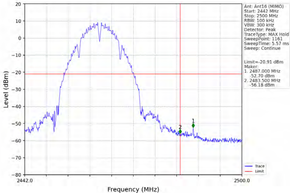
802.11b_HCH_2462MHz_Ant16 (MIMO)_NTNV
