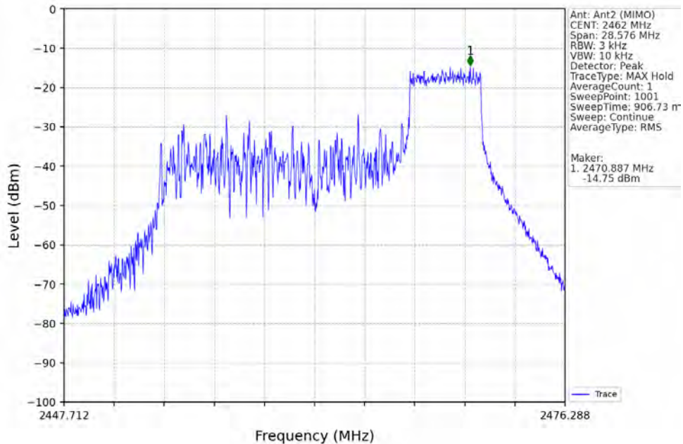
802.11be(EHT20)_HCH_2462MHz_RU52_Right_MIMO_NTNV
