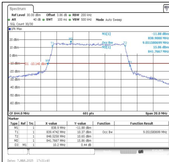
26(824-849)-10MHz-QPSK-26990-50RB#0-PASS
