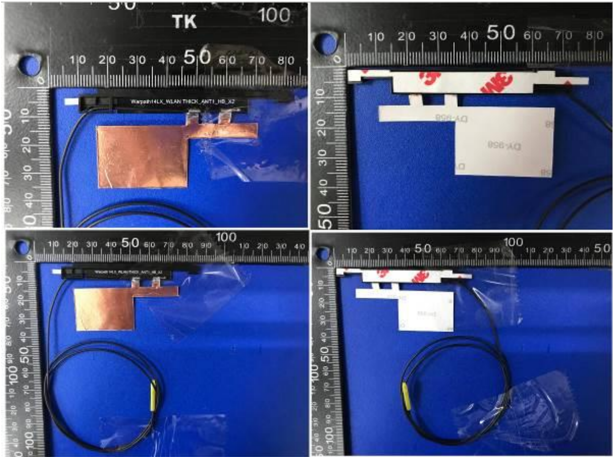
Tx1 (AUX) Antenna Photo:
