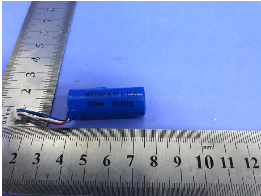
Photo 12 Battery parameter
