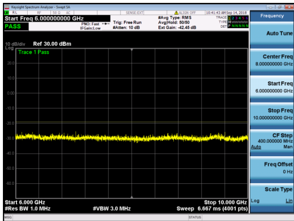
LTE20 Mid+NB IoT GB (Upper) 6000MHz-10000MHz
