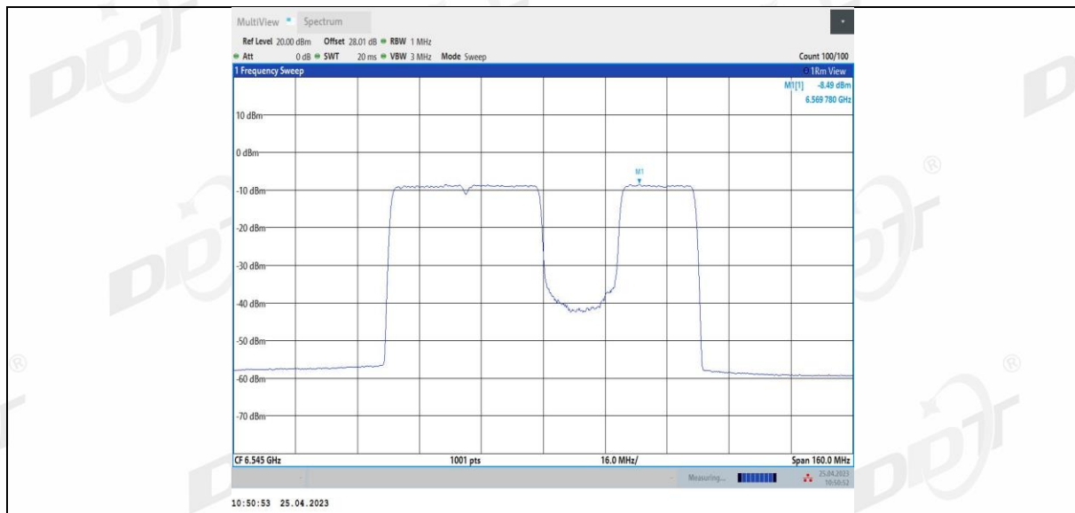
11BE80MIMO_Ant3_6545_484+242_4
