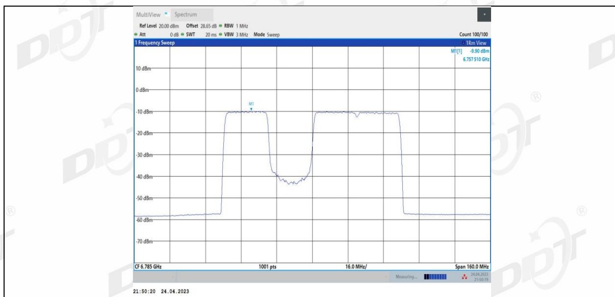
11BE80MIMO_Ant1_6785_484+242_3
