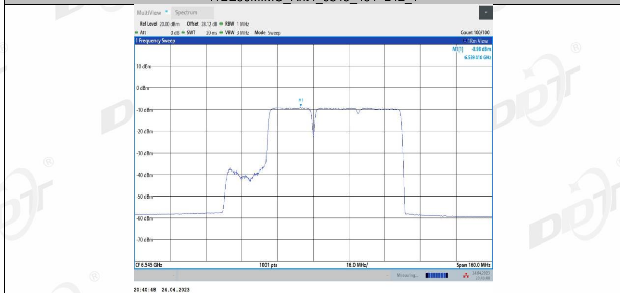
11BE80MIMO_Ant4_6545_484+242_2
