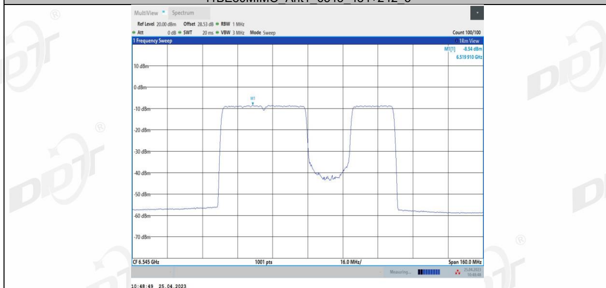
11BE80MIMO Ant1 6545 484+242 4
