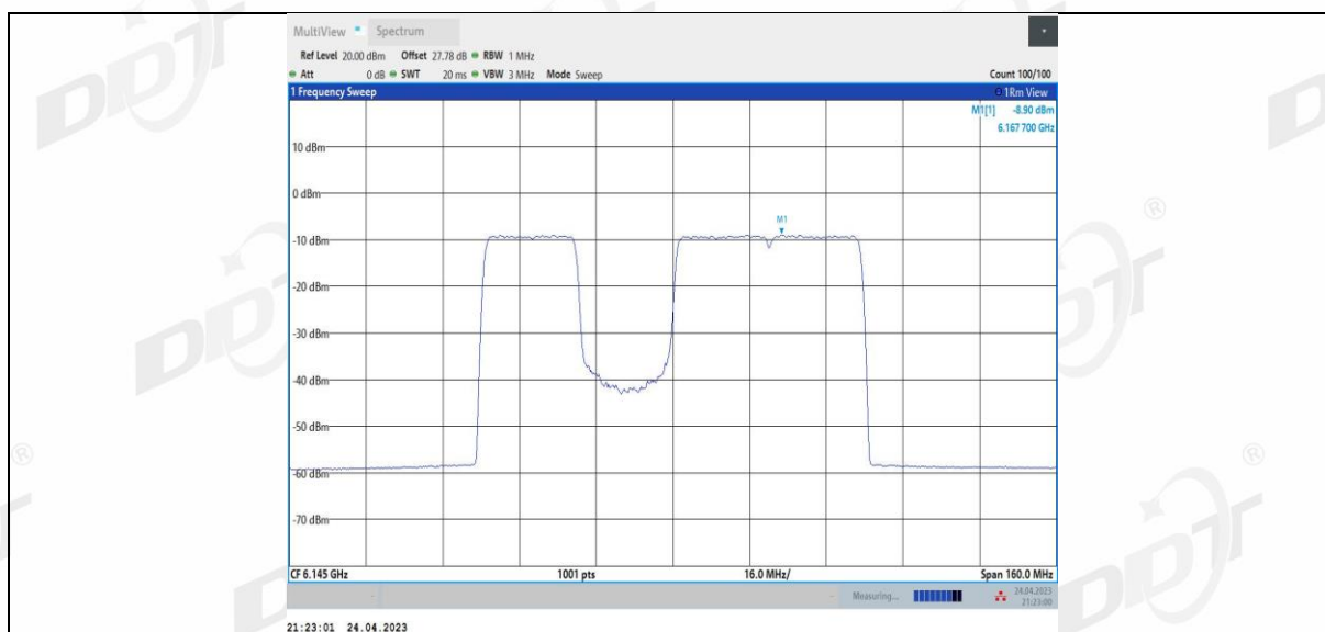
11BE80MIMO Ant1 6145 484+242 3
