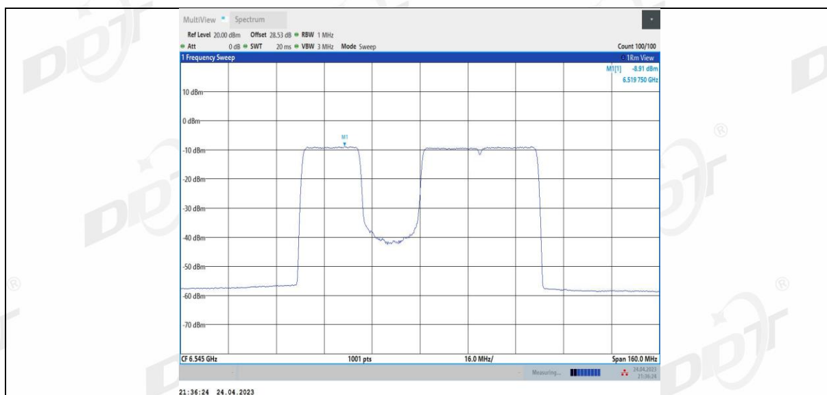
11BE80MIMO Ant1 6545 484+242 3
