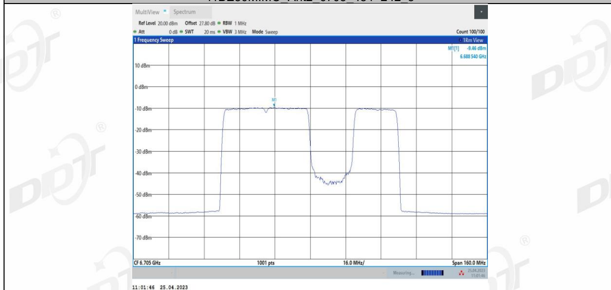
11BE80MIMO Ant2 6705 484+242_4
