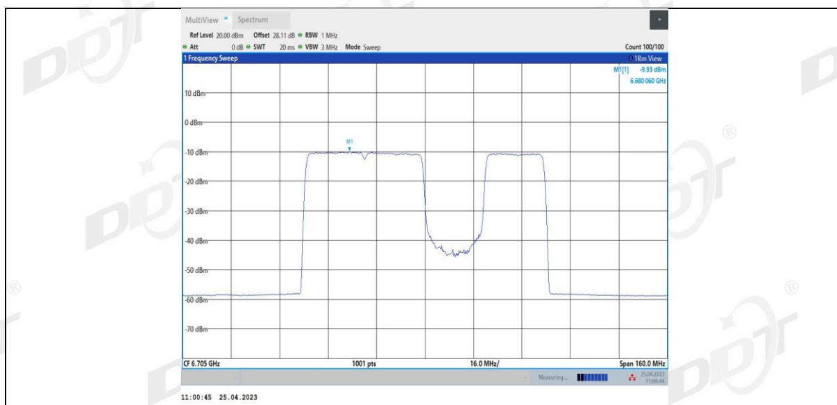
11BE80MIMO_Ant1_6705_484+242_4
