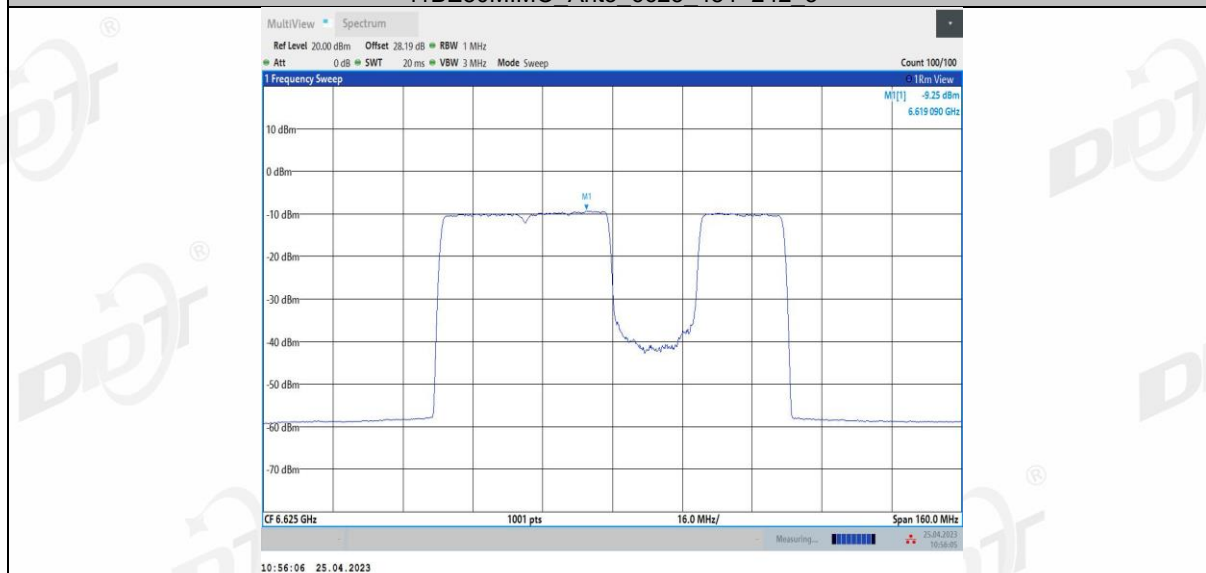
11BE80MIMO Ant3 6625 484+242_4
