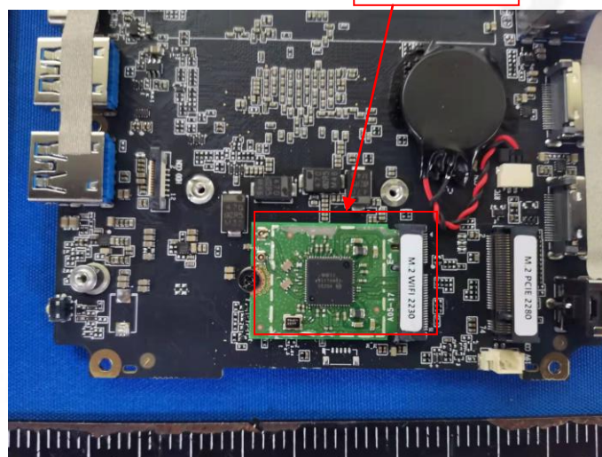
RF Module
