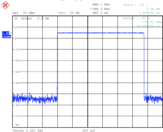
DH5_Hopping 2.908ms
