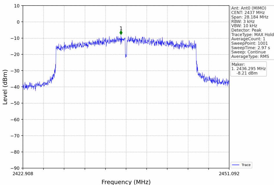
802.11ax(HEW20)_MCH_2437MHz_RU242_Left_Ant0 (MIMO)_NTNV
