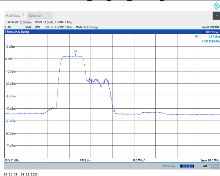
11AX40MIMO_Ant1_5510_242Tone_RU61
