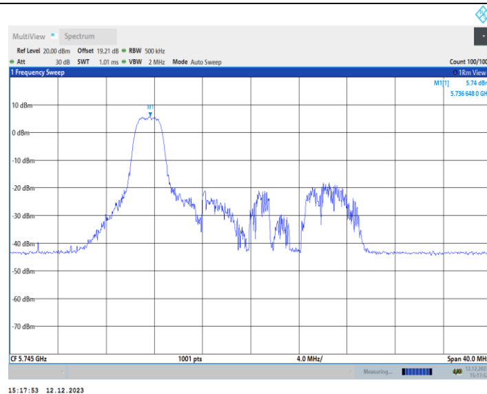
11AX20MIMO_Ant2_5745_52Tone_RU37
