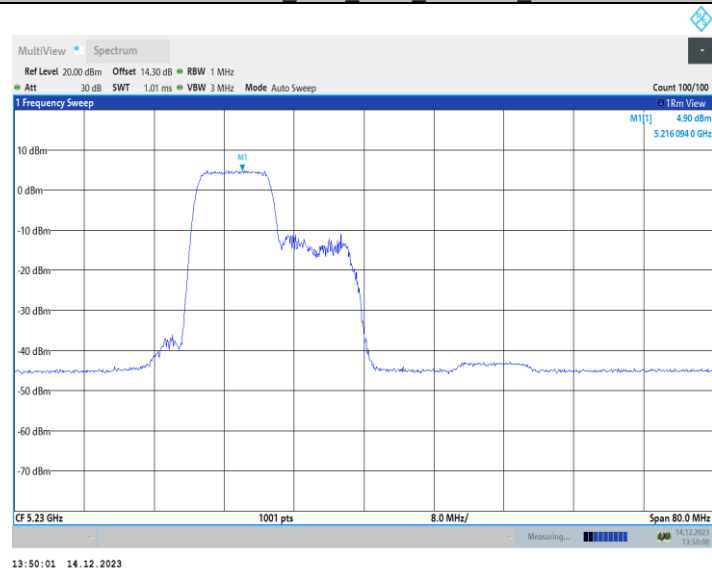
11AX40MIMO_Ant1_5230_242Tone_RU61
