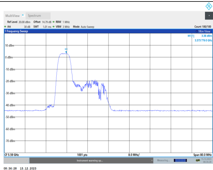
11AX40MIMO_Ant2_5590_106Tone_RU53
