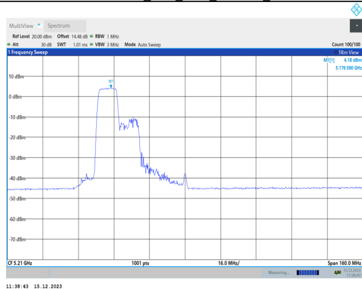
11AX80MIMO_Ant2_5210_242Tone_RU64
