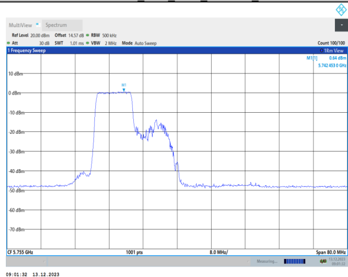
11AX40MIMO_Ant2_5755_242Tone_RU61
