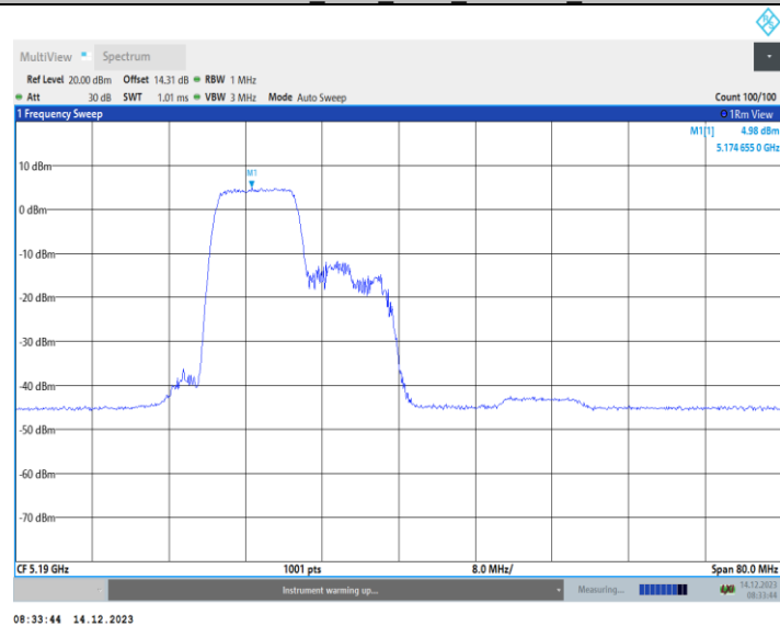
11AX40MIMO_Ant1_5190_242Tone_RU61
