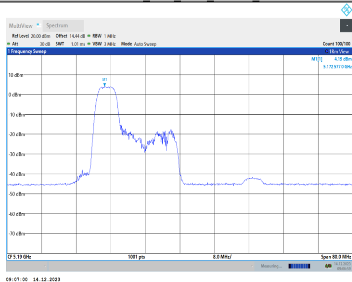
11AX40MIMO_Ant2_5190_106Tone_RU53
