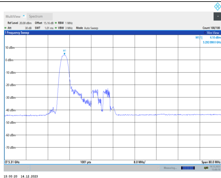
11AX40MIMO_Ant1_5310_52Tone_RU37
