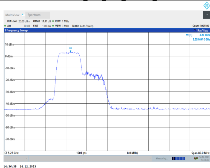
11AX40MIMO_Ant2_5270_242Tone_RU61
