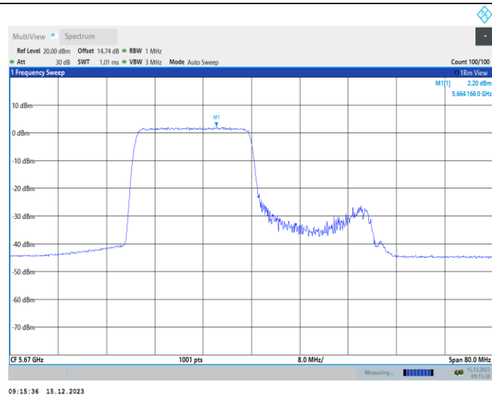
11AX40MIMO_Ant2_5670_26Tone_RU0
