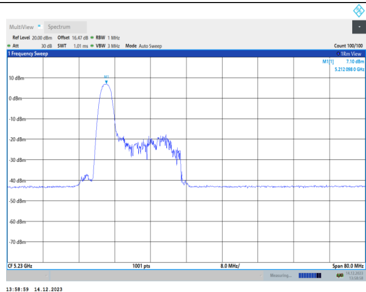
11AX40MIMO_Ant2_5230_52Tone_RU37
