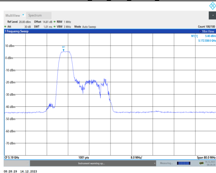
11AX40MIMO_Ant1_5190_106Tone_RU53
