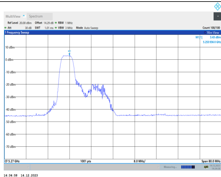
11AX40MIMO_Ant2_5270_106Tone_RU53
