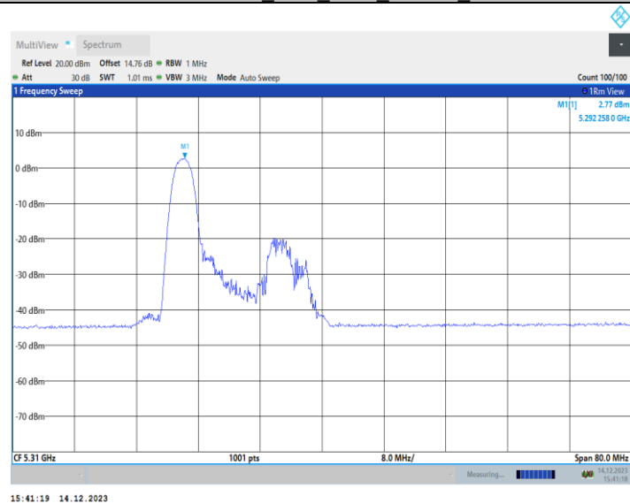
11AX40MIMO_Ant2_5310_52Tone_RU37
