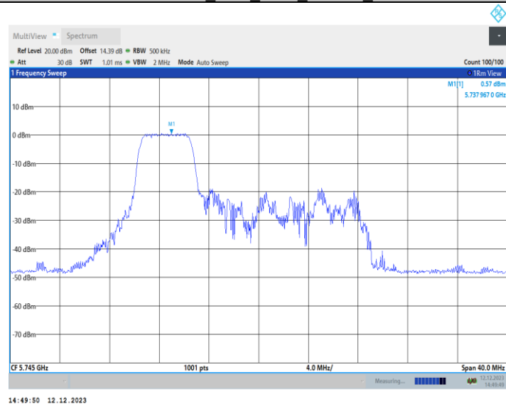
11AX20MIMO_Ant1_5745_106Tone_RU53
