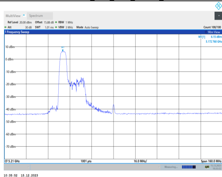
11AX80MIMO_Ant1_5210_106Tone_RU53
