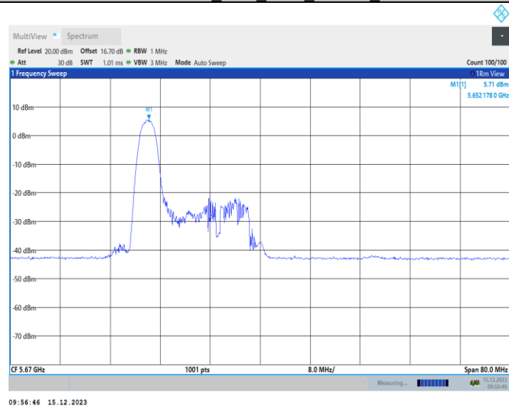
11AX40MIMO_Ant2_5670_52Tone_RU37
