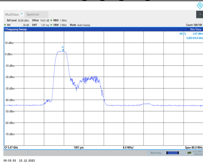
11AX40MIMO_Ant1_5670_106Tone_RU53
