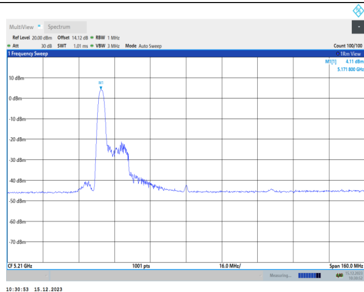
11AX80MIMO_Ant1_5210_52Tone_RU37
