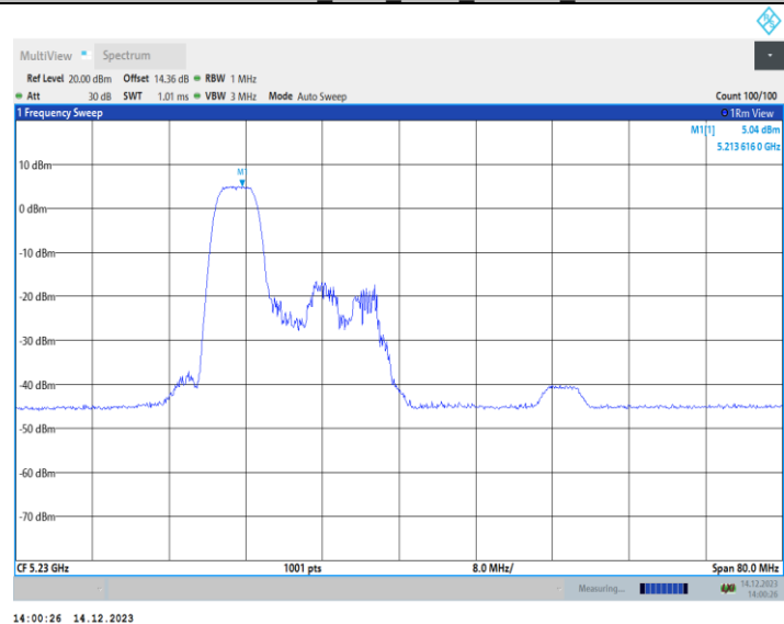
11AX40MIMO_Ant2_5230_106Tone_RU53
