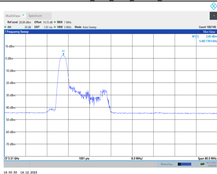
11AX40MIMO Ant1 5510 52Tone RU37
