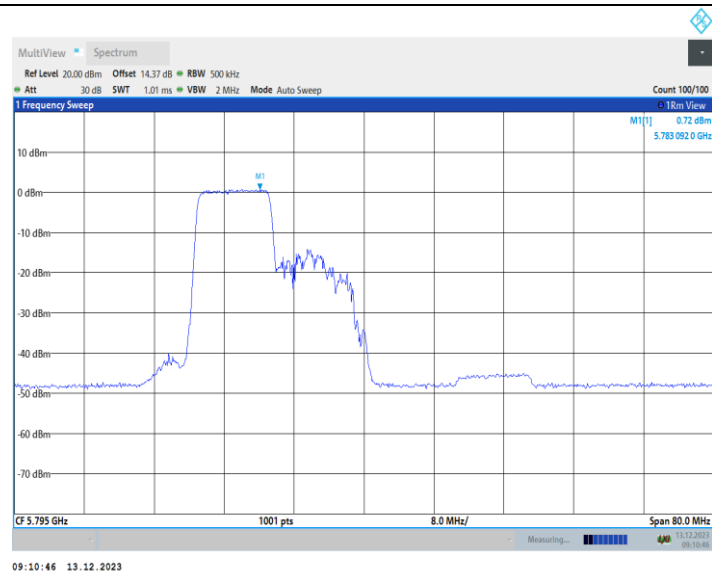
11AX40MIMO_Ant1_5795_242Tone_RU61
