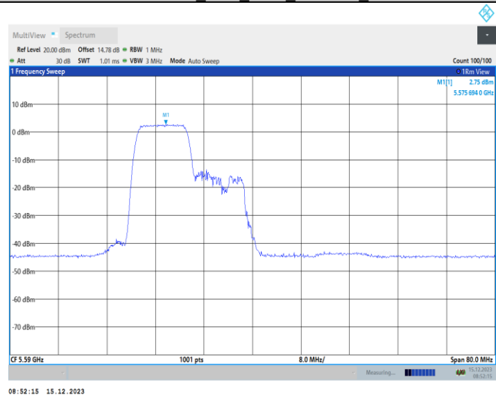
11AX40MIMO_Ant2_5590_242Tone_RU61
