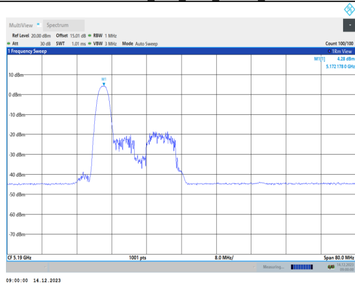
11AX40MIMO_Ant2_5190_52Tone_RU37
