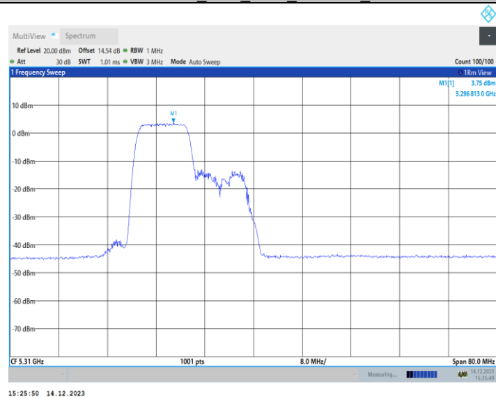
11AX40MIMO_Ant1_5310_242Tone_RU61
