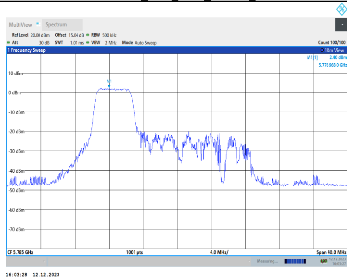
11AX20MIMO_Ant2_5785_106Tone_RU53
