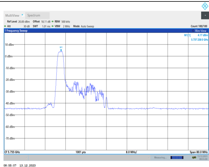
11AX40MIMO_Ant2_5755_52Tone_RU37
