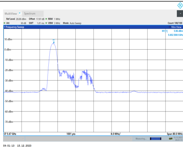
11AX40MIMO_Ant1_5670_52Tone_RU37
