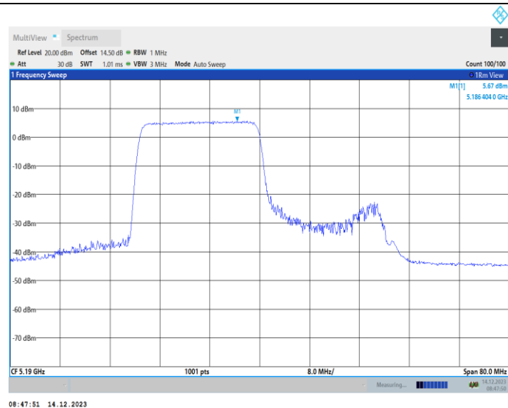
11AX40MIMO_Ant2_5190_26Tone_RU0
