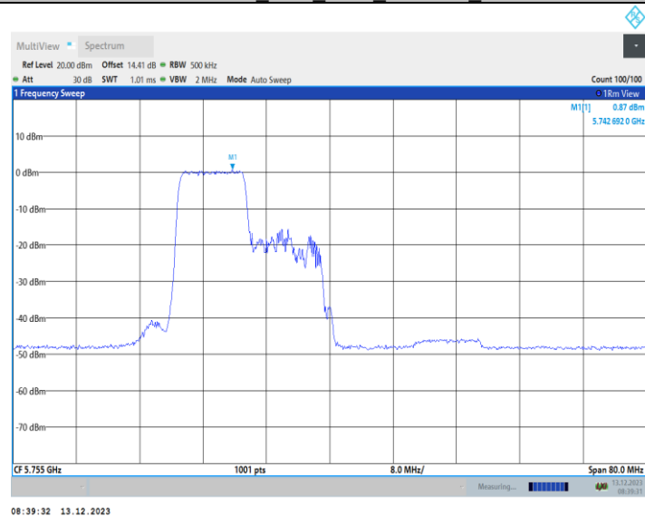
11AX40MIMO Ant1 5755 242Tone RU61
