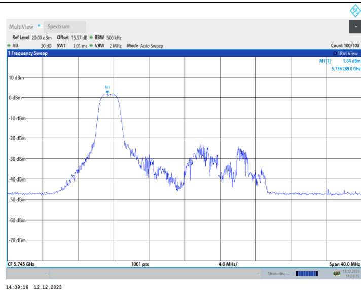
11AX20MIMO_Ant1_5745_52Tone_RU37
