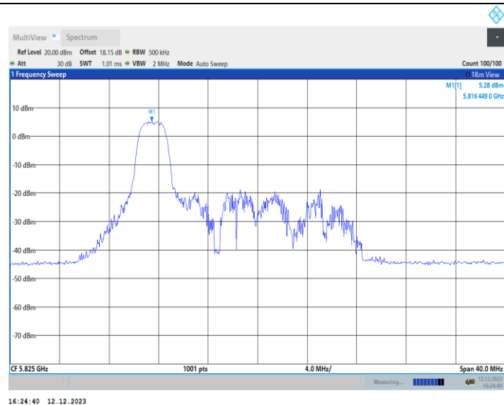
11AX20MIMO_Ant1_5825_52Tone_RU37
