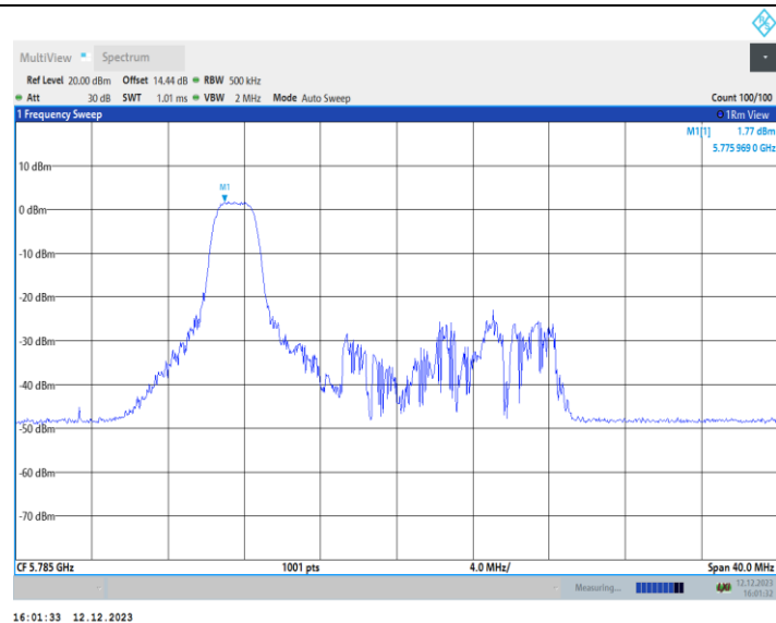
11AX20MIMO_Ant2_5785_52Tone_RU37
