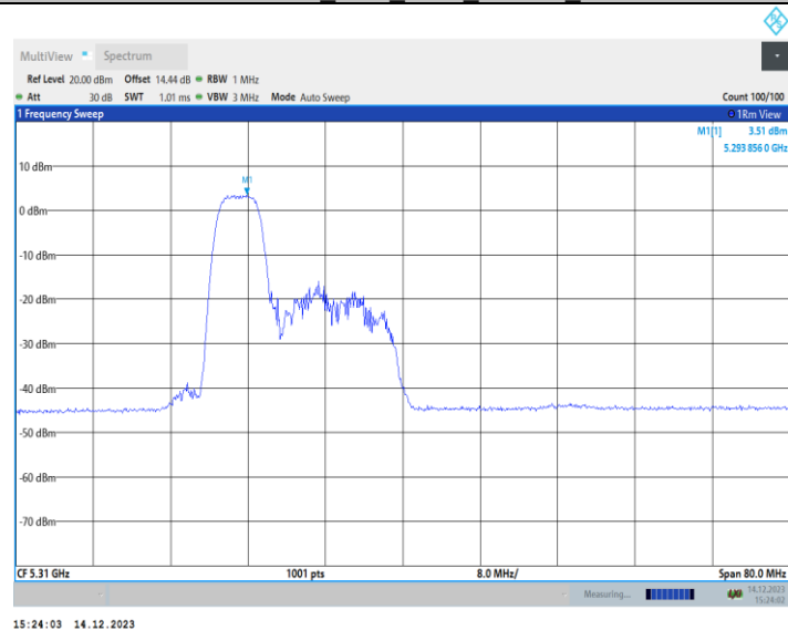
11AX40MIMO_Ant1_5310_106Tone_RU53
