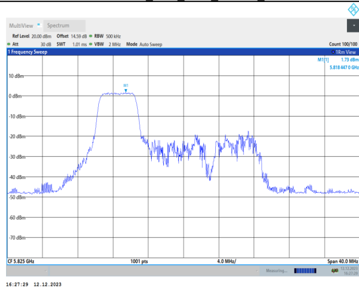
11AX20MIMO_Ant1_5825_106Tone_RU53
