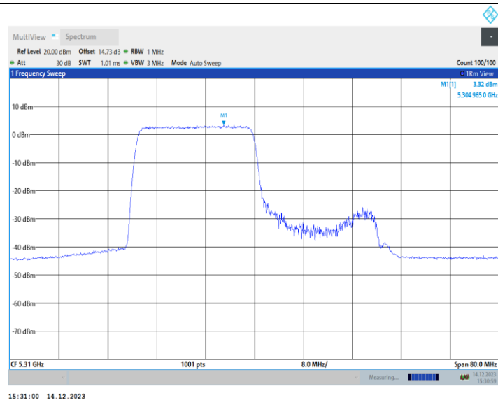
11AX40MIMO_Ant2_5310_26Tone_RU0
