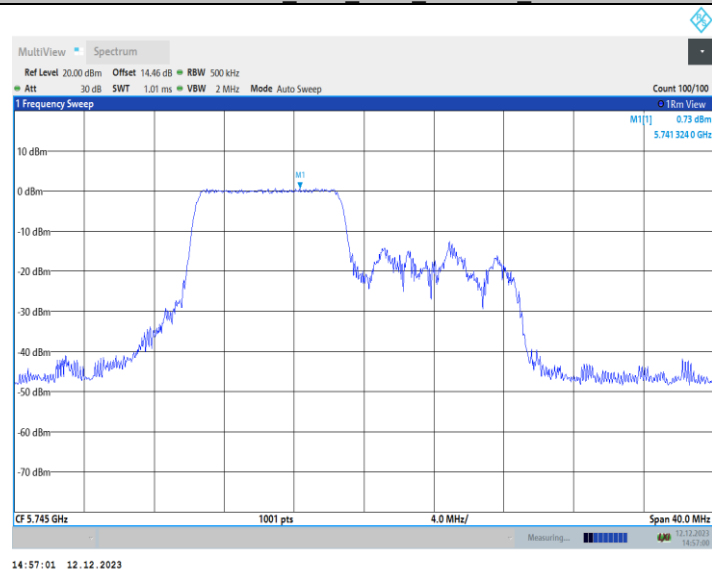
11AX20MIMO_Ant2_5745_26Tone_RU0
