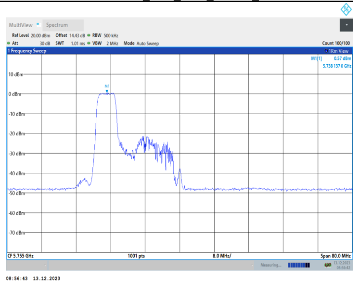
11AX40MIMO_Ant2_5755_106Tone_RU53
