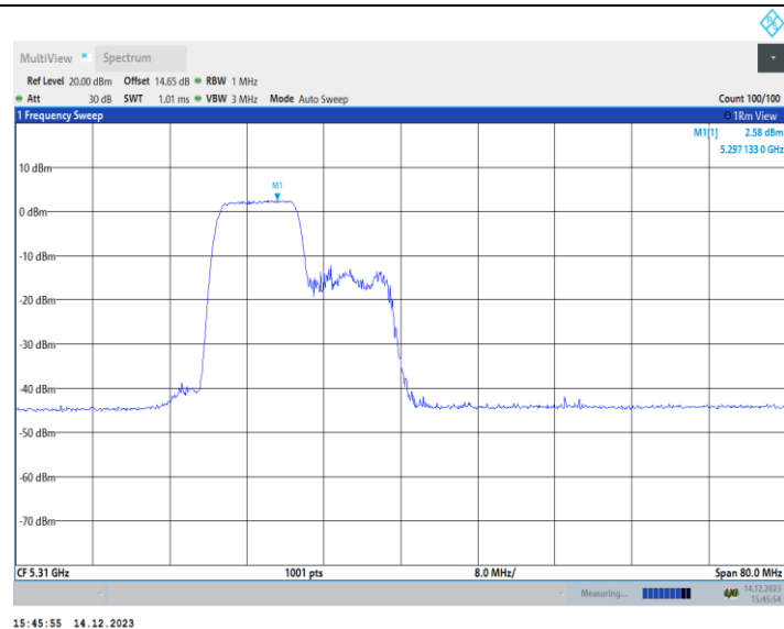
11AX40MIMO Ant2 5310 242Tone RU61
