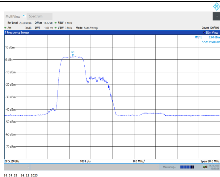
11AX40MIMO Ant1 5590 242Tone RU61
