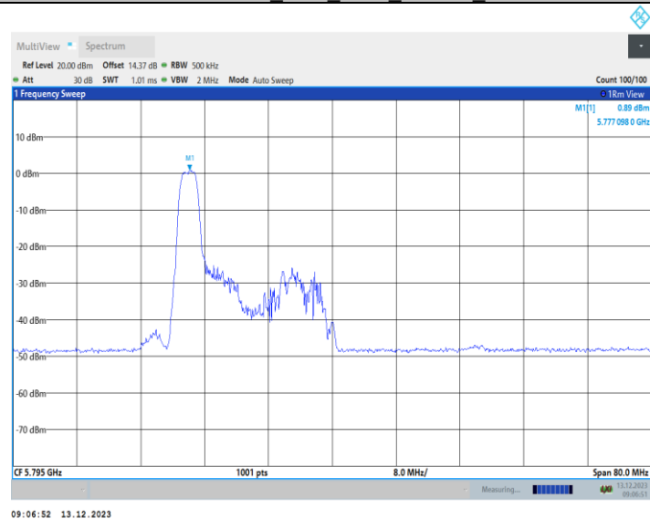
11AX40MIMO_Ant1_5795_52Tone_RU37
