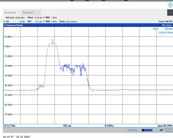
11AX40MIMO_Ant1_5270_106Tone_RU53
