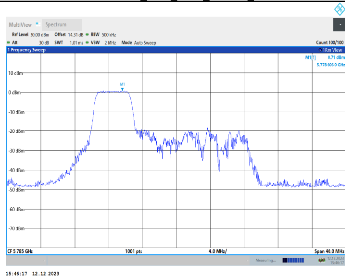
11AX20MIMO_Ant1_5785_106Tone_RU53
