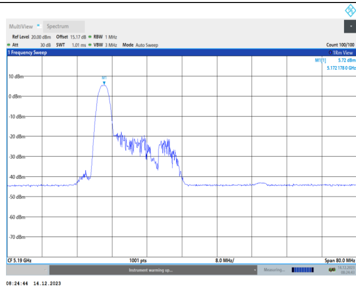
11AX40MIMO_Ant1_5190_52Tone_RU37
