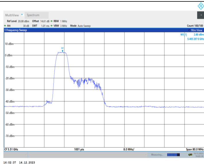
11AX40MIMO_Ant1_5510_106Tone_RU53
