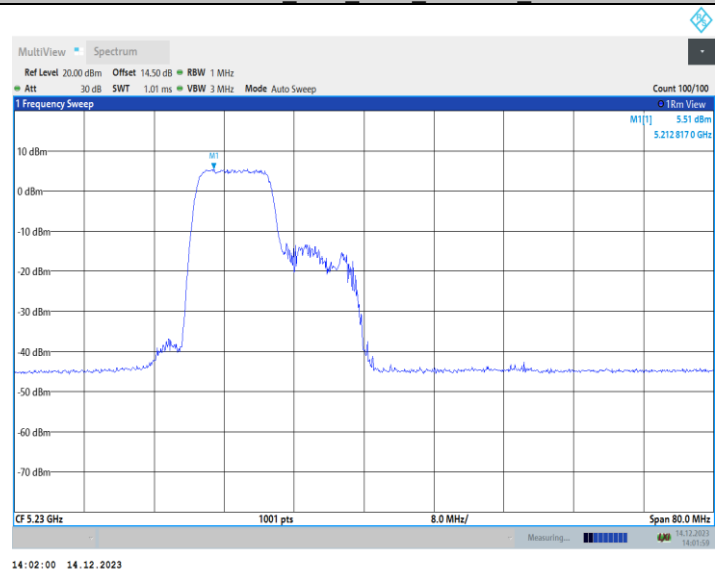
11AX40MIMO_Ant2_5230_242Tone_RU61
