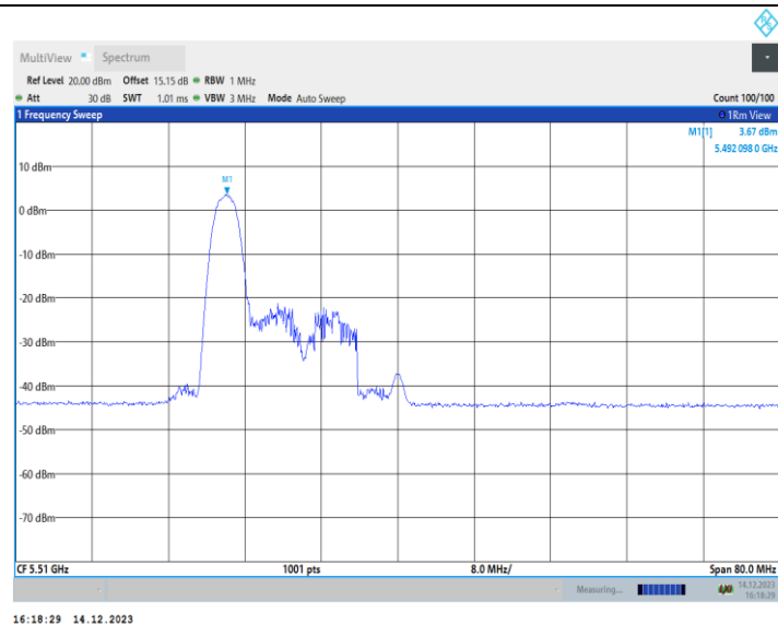
11AX40MIMO_Ant2_5510_52Tone_RU37
