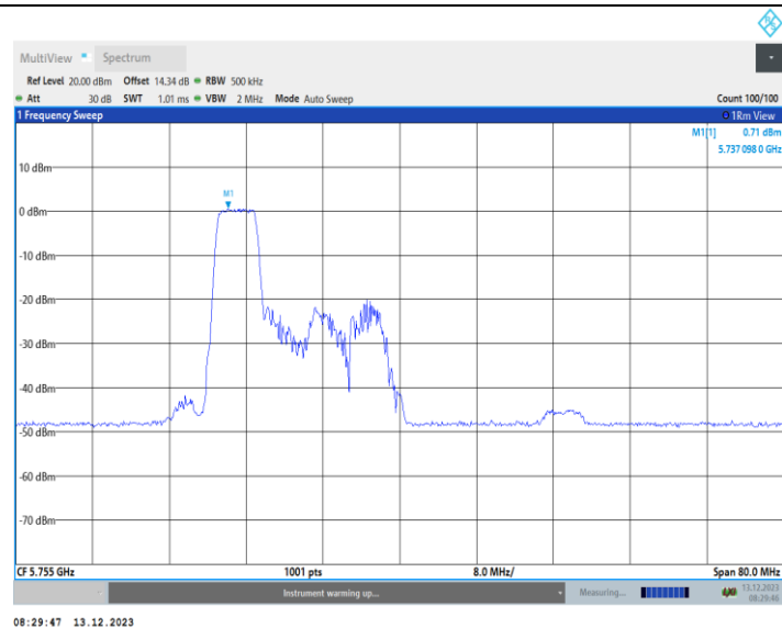
11AX40MIMO Ant1 5755 106Tone RU53
