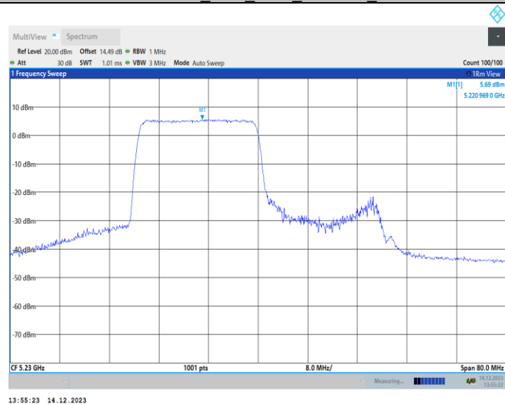
11AX40MIMO_Ant2_5230_26Tone_RU0
