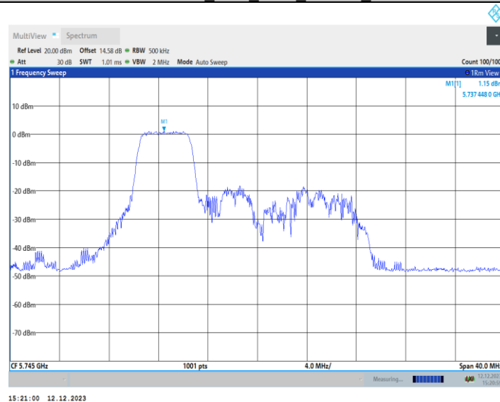
11AX20MIMO_Ant2_5745_106Tone_RU53
