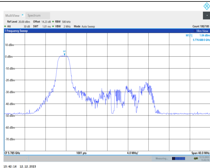
11AX20MIMO_Ant1_5785_52Tone_RU37
