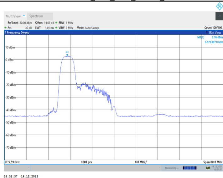
11AX40MIMO_Ant1_5590_106Tone_RU53
