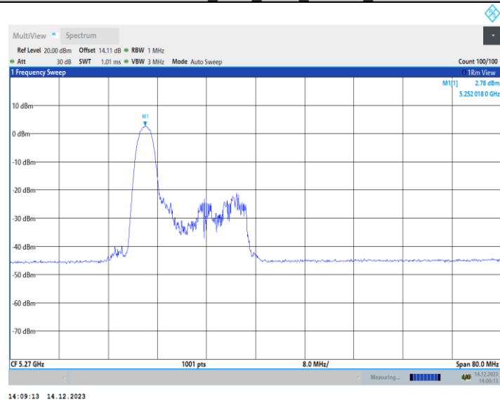
11AX40MIMO_Ant1_5270_52Tone_RU37
