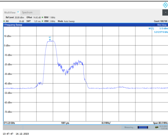
11AX40MIMO_Ant1_5230_106Tone_RU53
