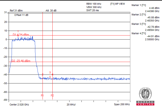
Chain 1 : CH 9 Band edge
