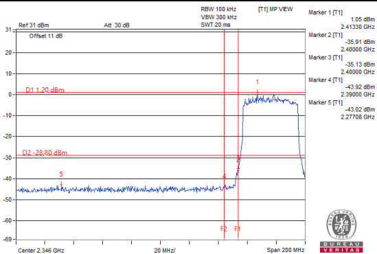
Chain 1 : CH 3 Band edge
