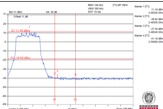
Chain 1 : CH 11 Band edge
